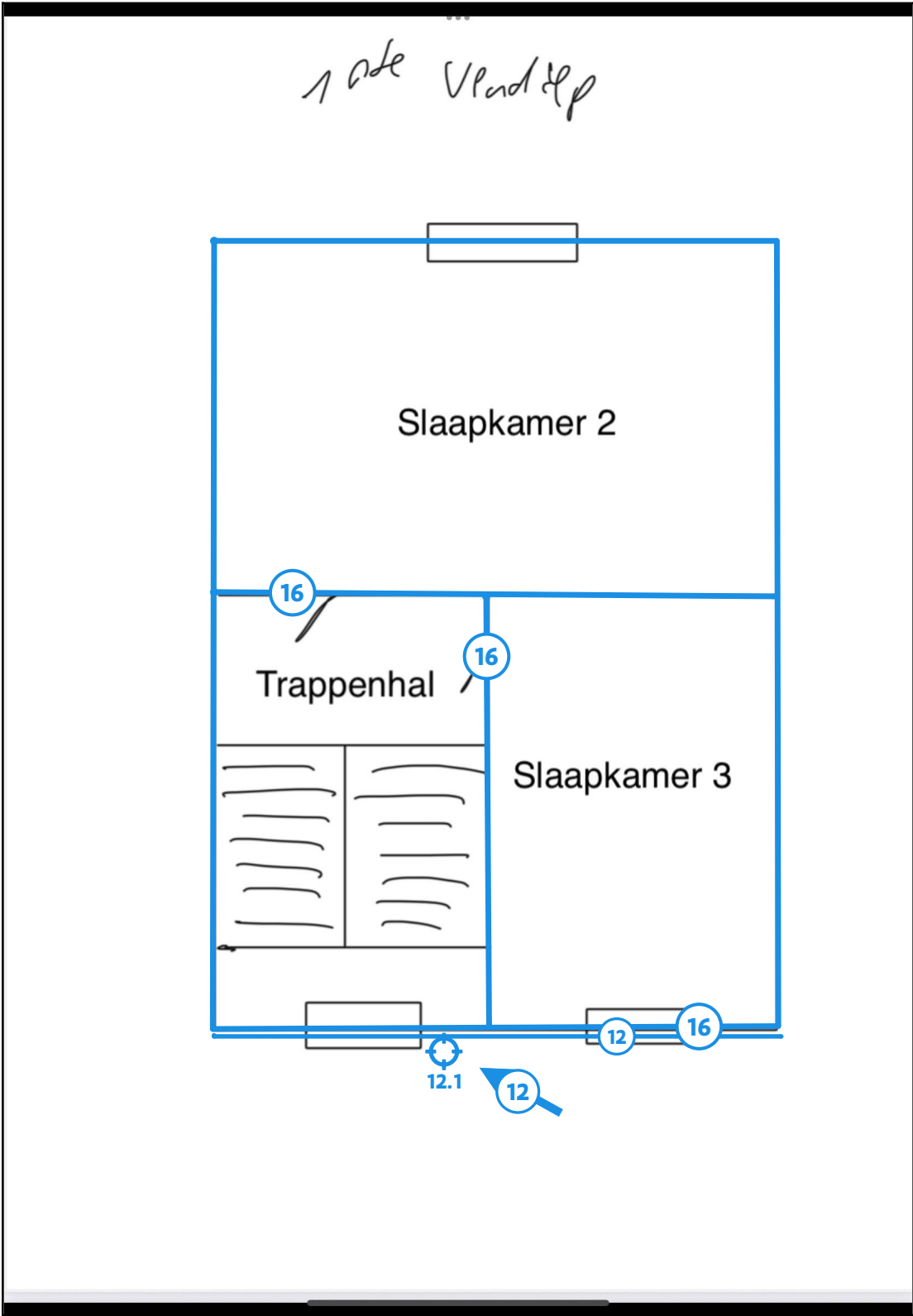
Legende van plan 1.6: 1ste verdiep wanden
