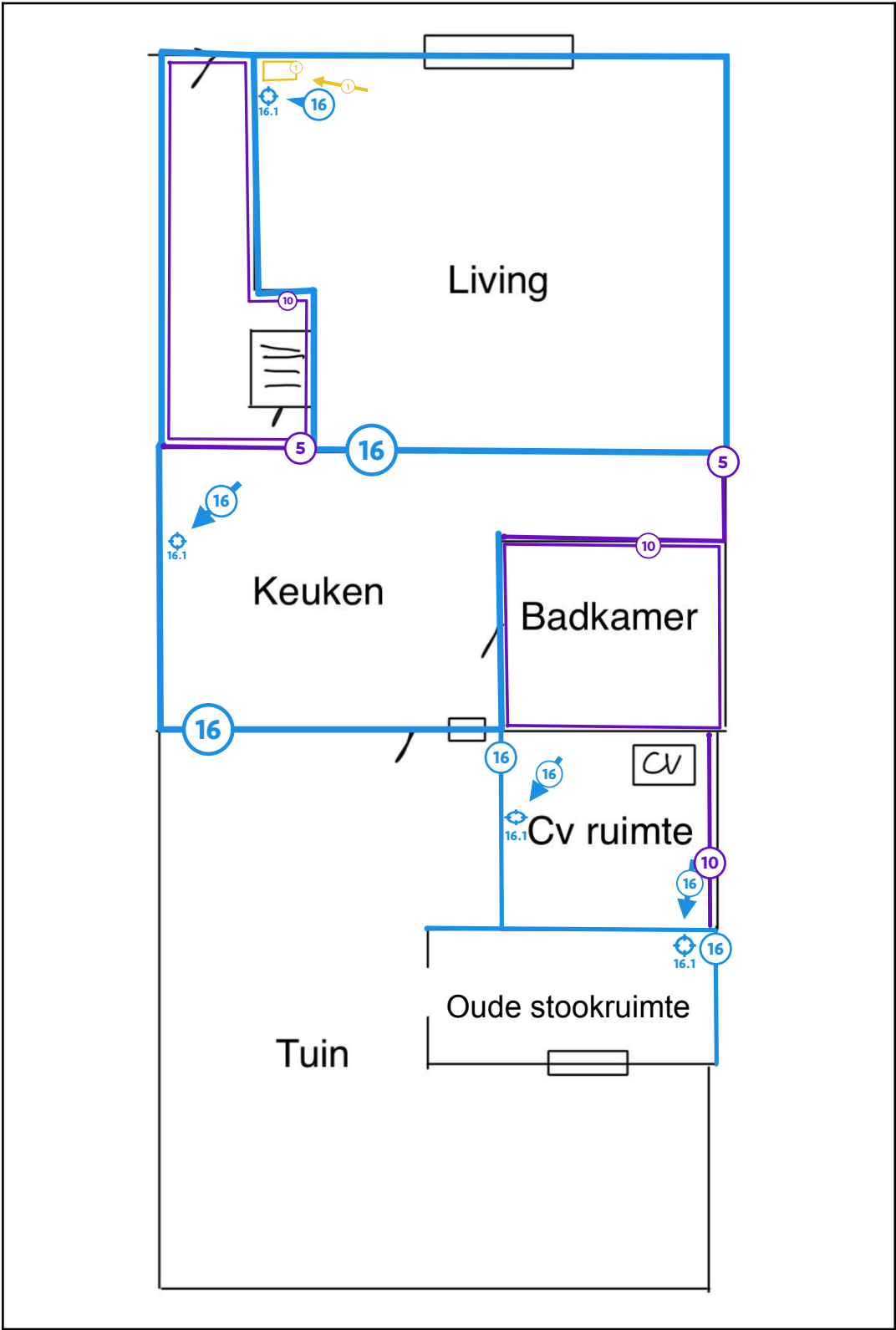
Legende van plan 1.9: Gelijkvloers wanden
