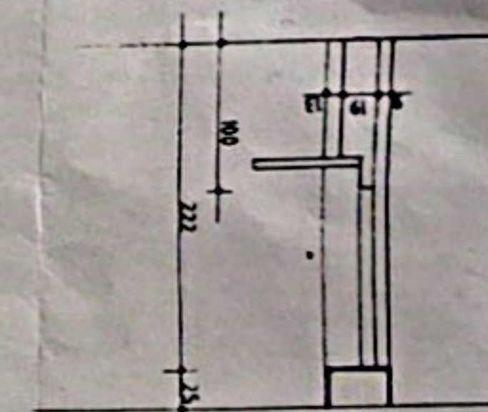
COUPE A IDÉAL SDB 11
