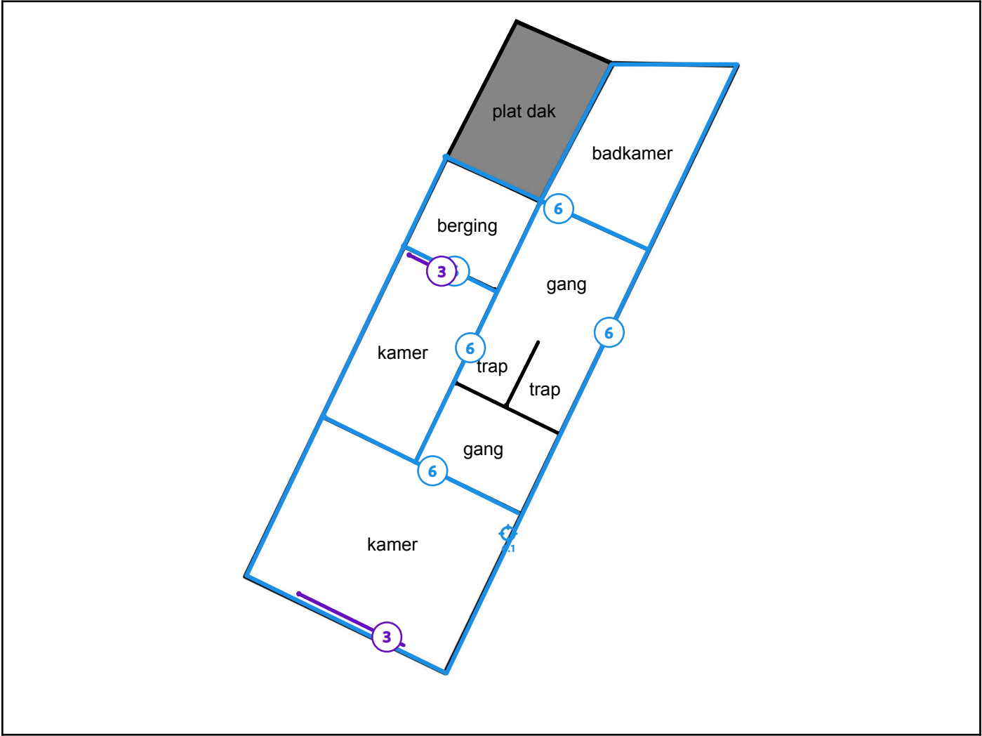
Legende van plan 1.3: Eerste verdiep; pleister wand en radiators
