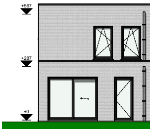
Achtergevel
