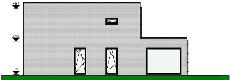
Rechtergevel
