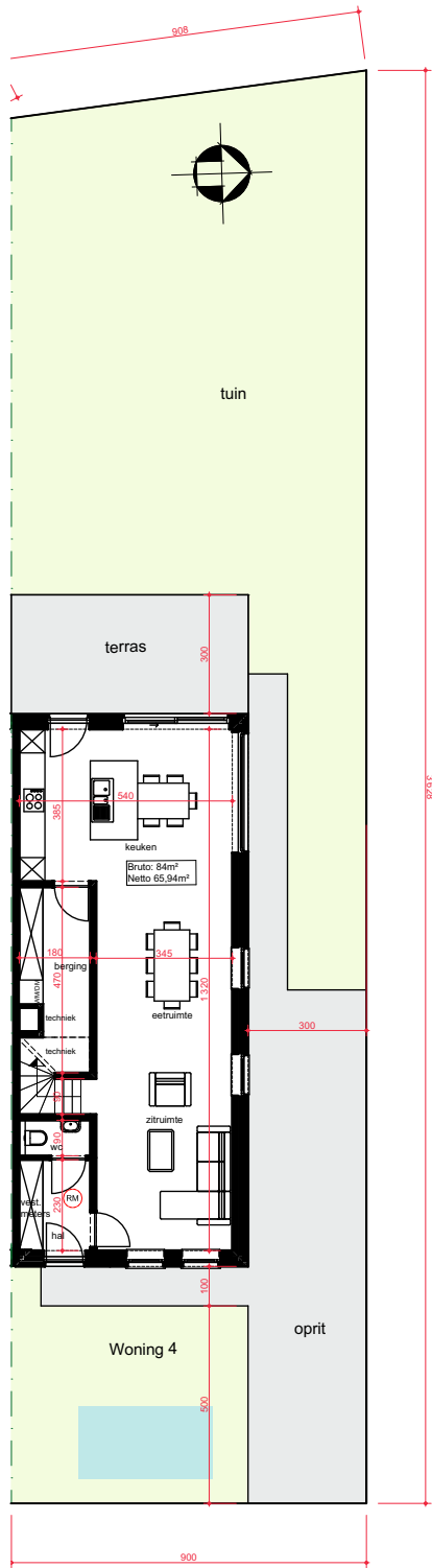
Gelijkvloers
