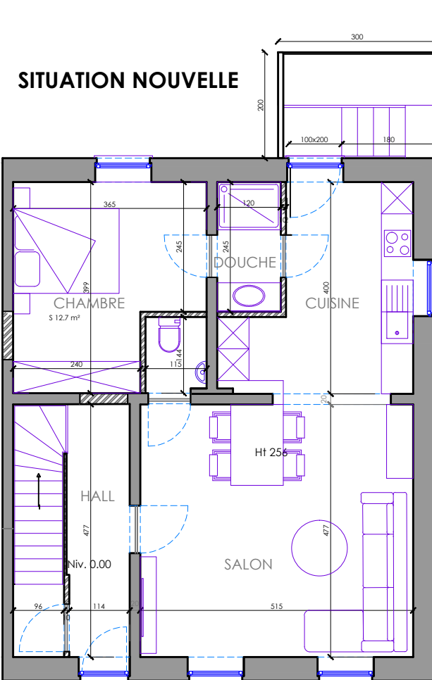
REZ DE CHAUSSEE Studio
