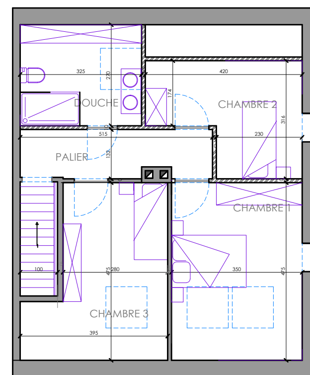
2ème ETAGE Duplex
