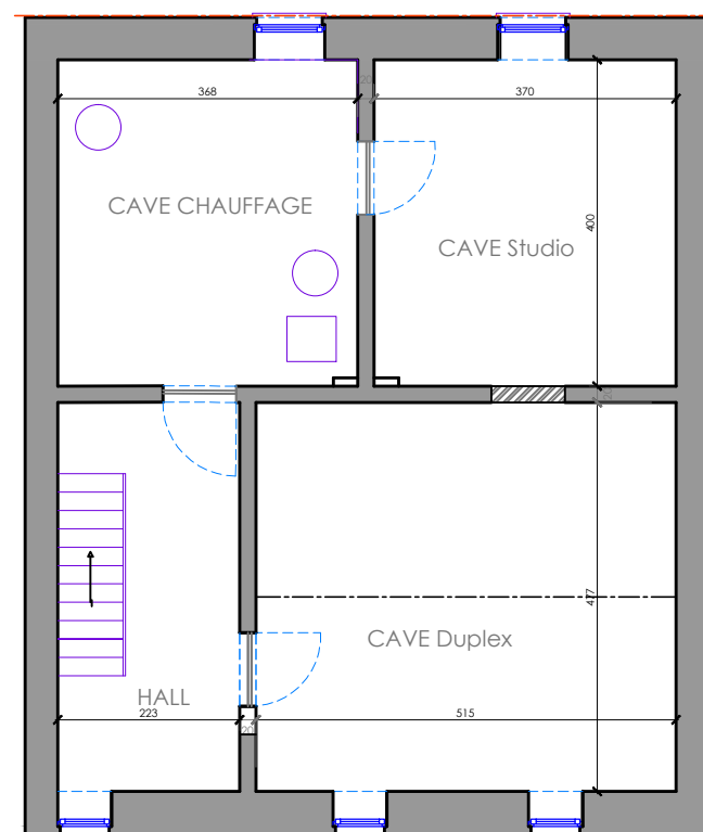
SOUS SOL
