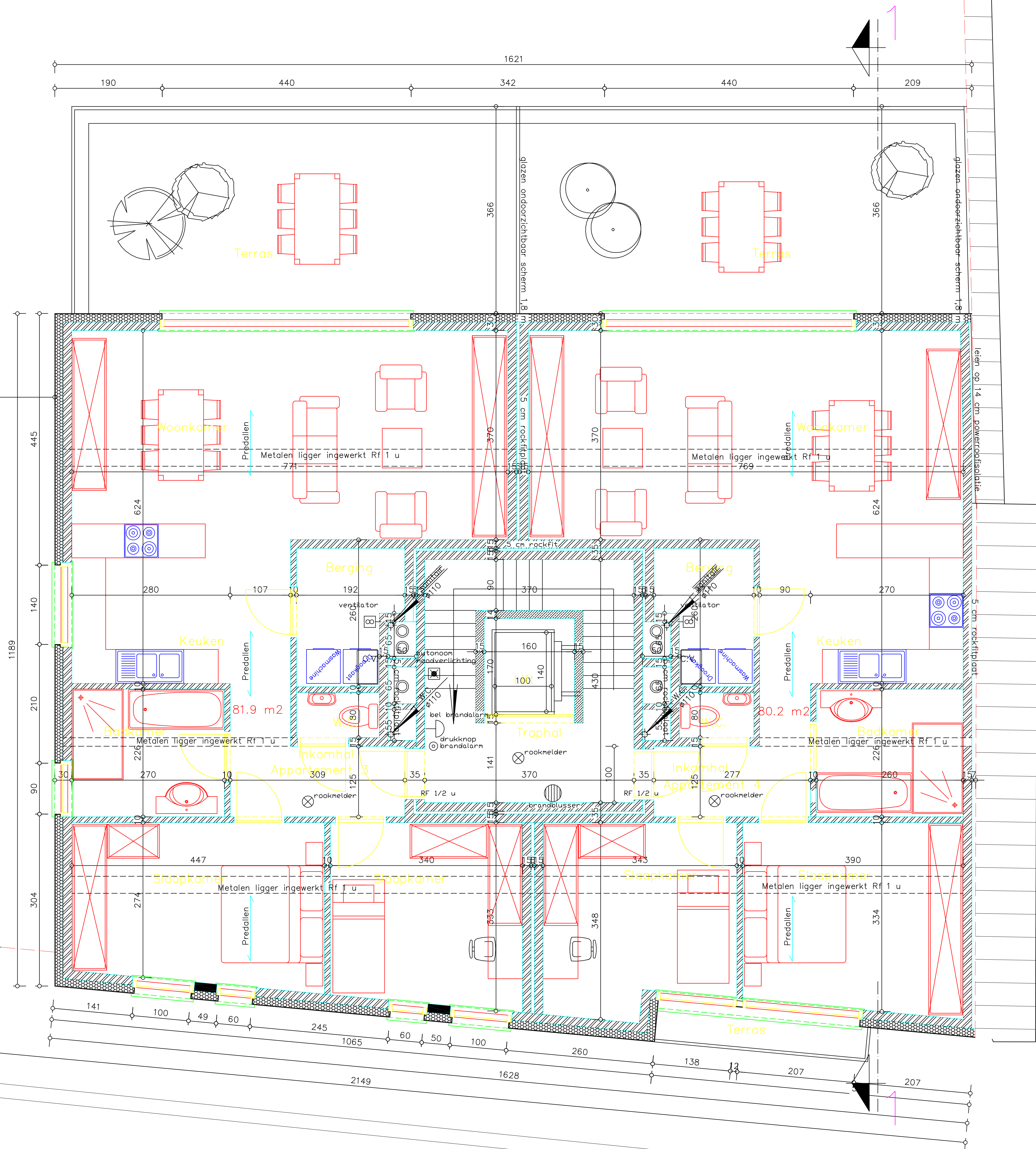
Verdiepingsplan 1°
