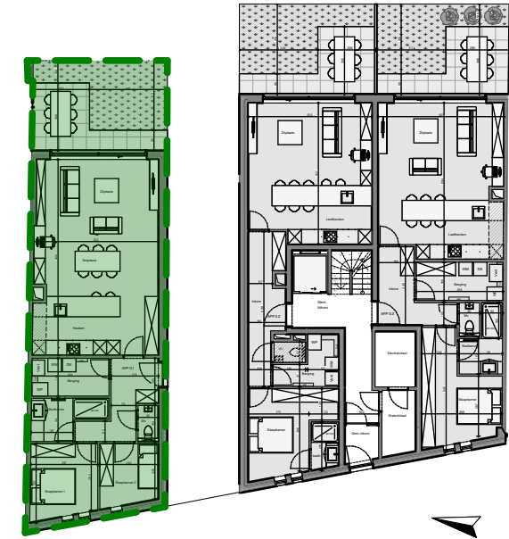
GRONDPLAN
