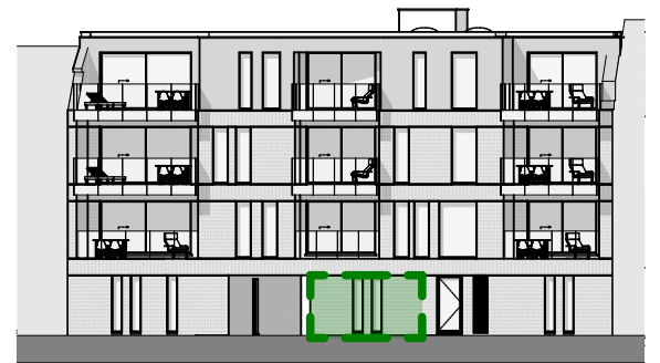
VOORGEVEL
