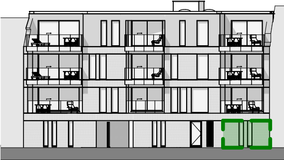
VOORGEVEL
