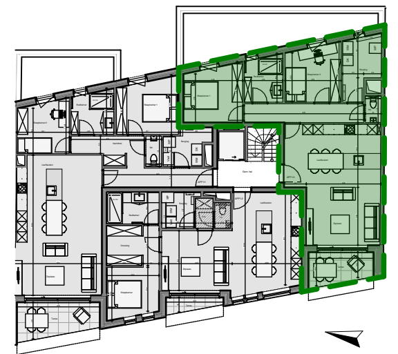
GRONDPLAN
