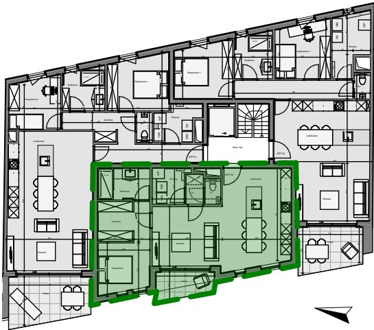
GRONDPLAN
