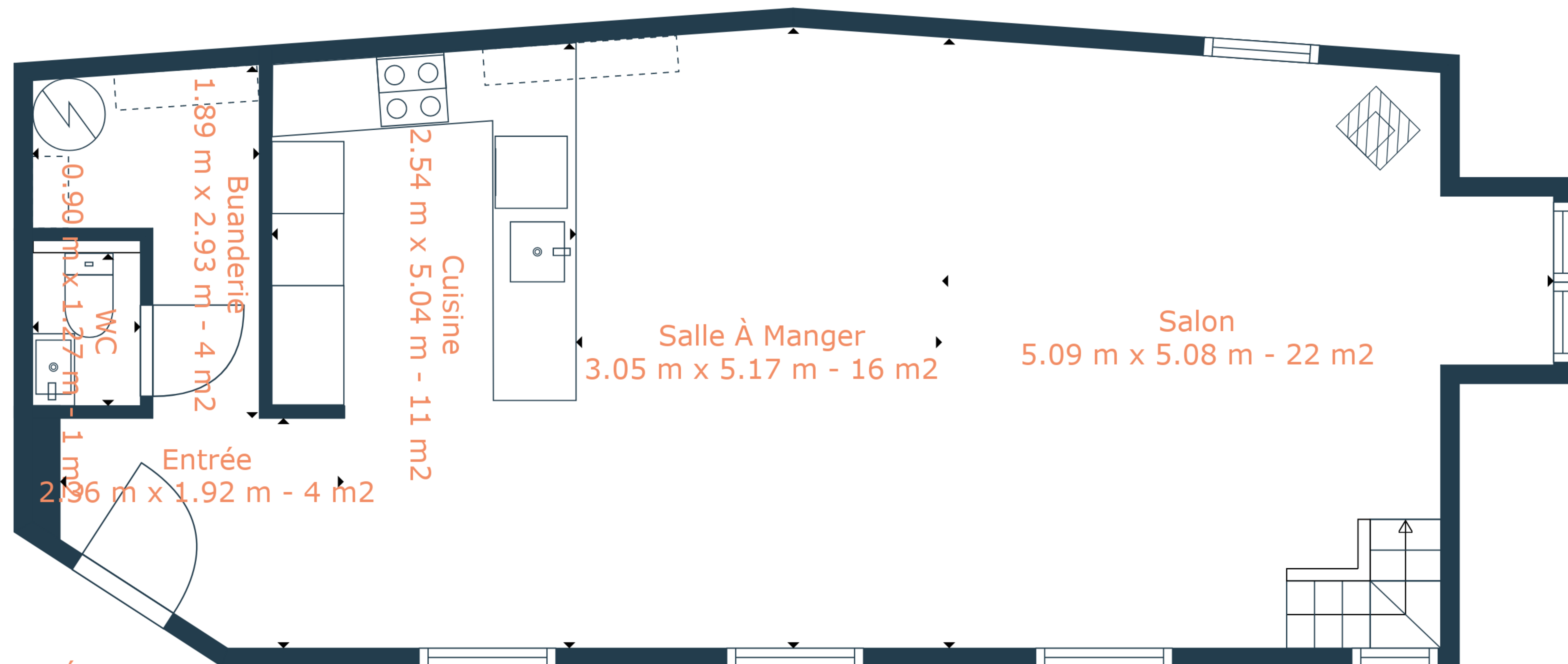
1er Étage
