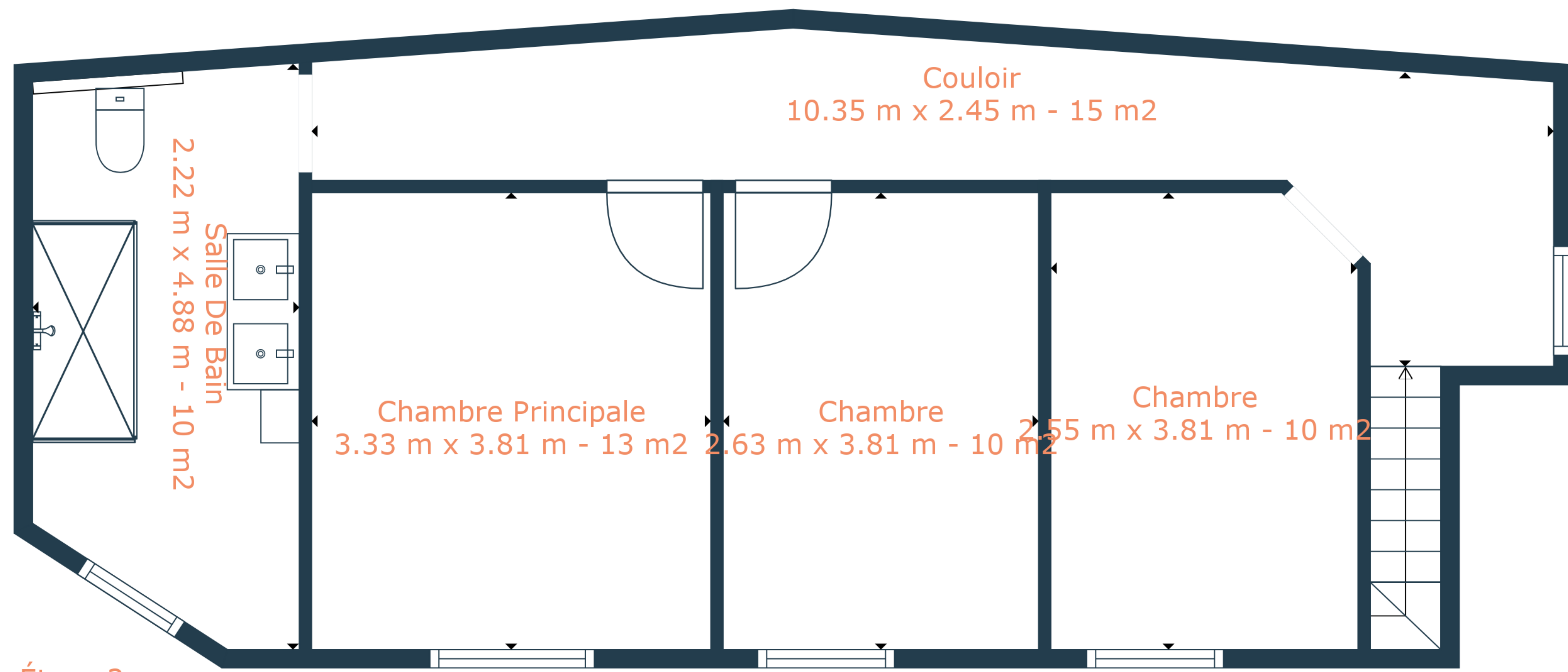
Étage 2
