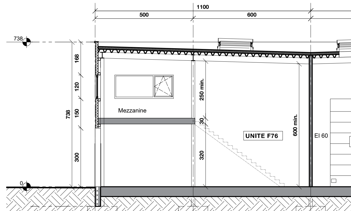
COUPE
