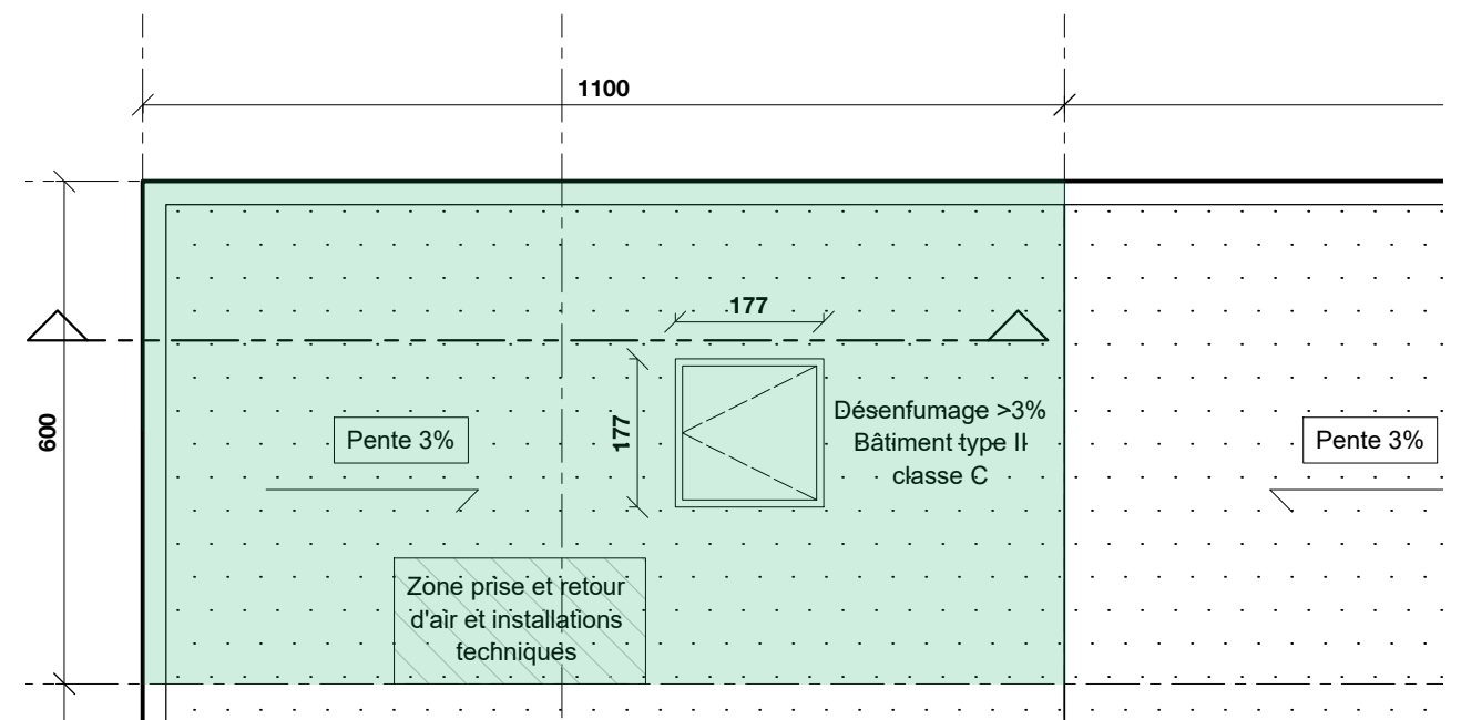
VUE EN PLAN TOITURE
