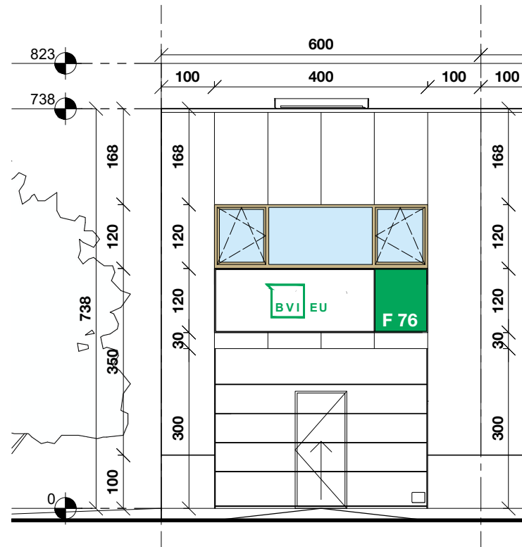
FACADE AVANT
