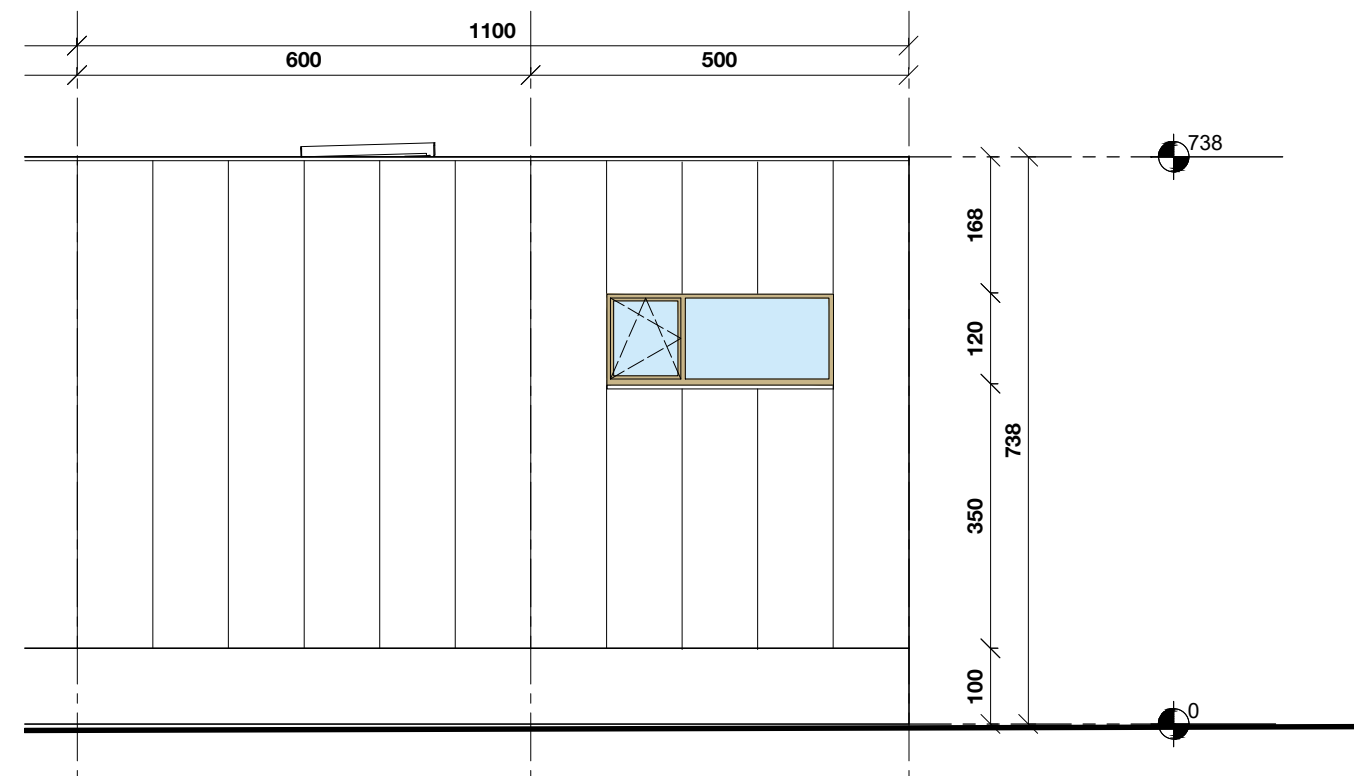
FACADE LATÉRALE
