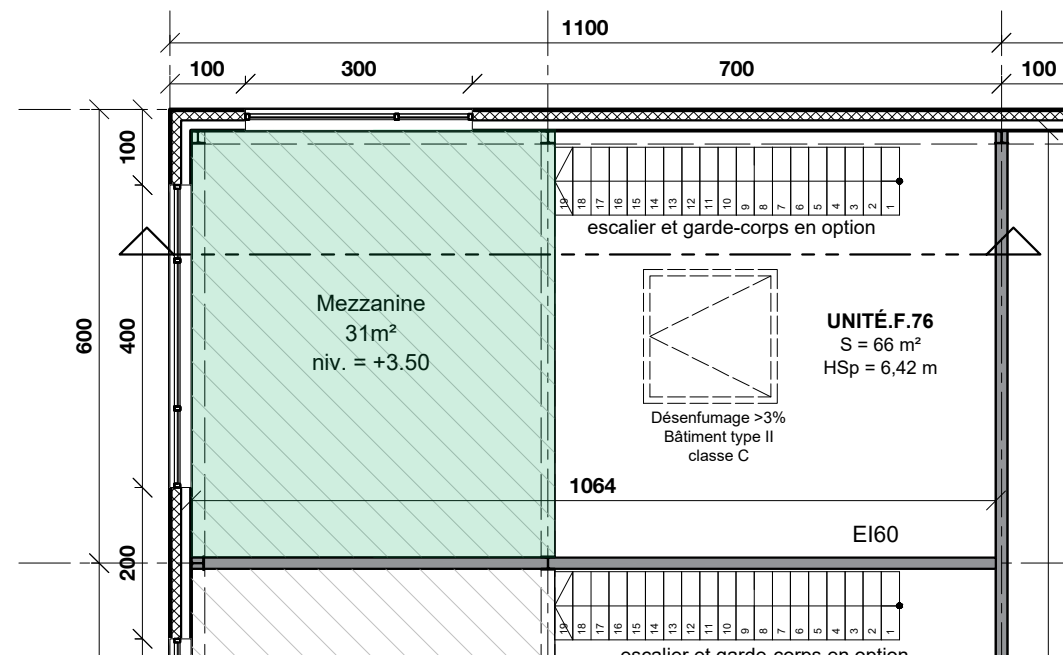
VUE EN PLAN R+1
