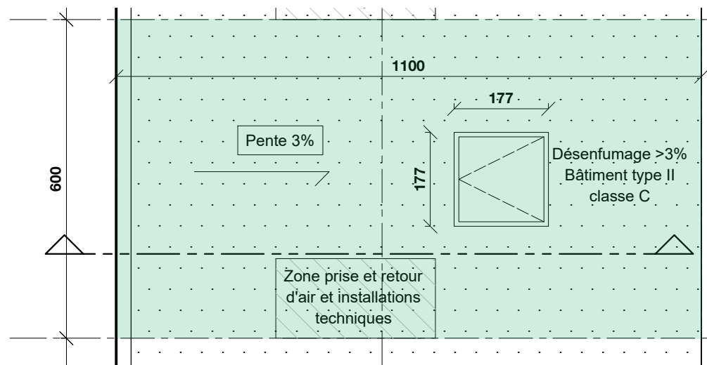
VUE EN PLAN TOITURE
