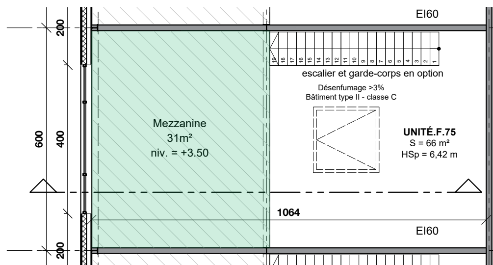
VUE EN PLAN R+1
