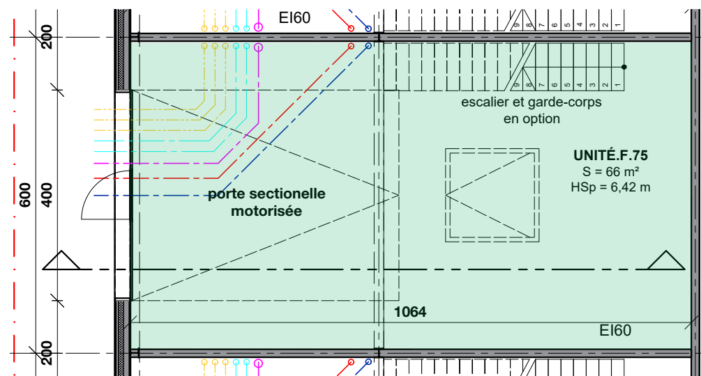
VUE EN PLAN RDC
