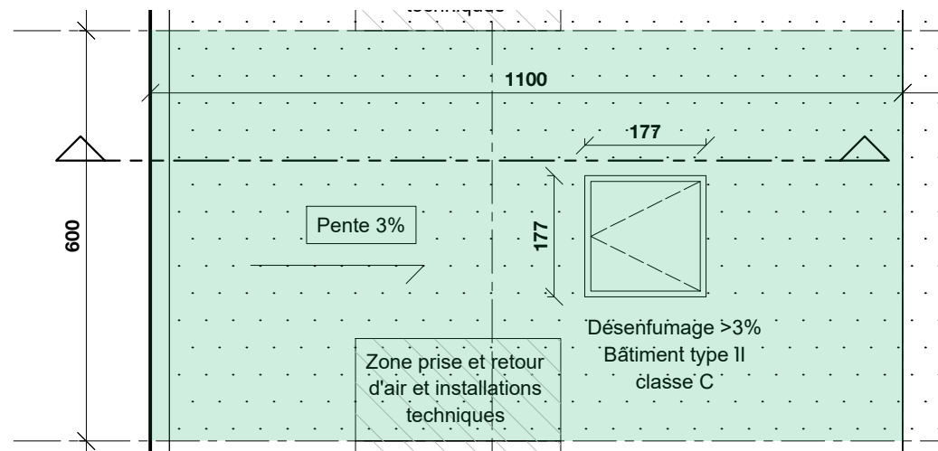
VUE EN PLAN TOITURE
