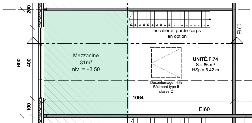
VUE EN PLAN R+1
