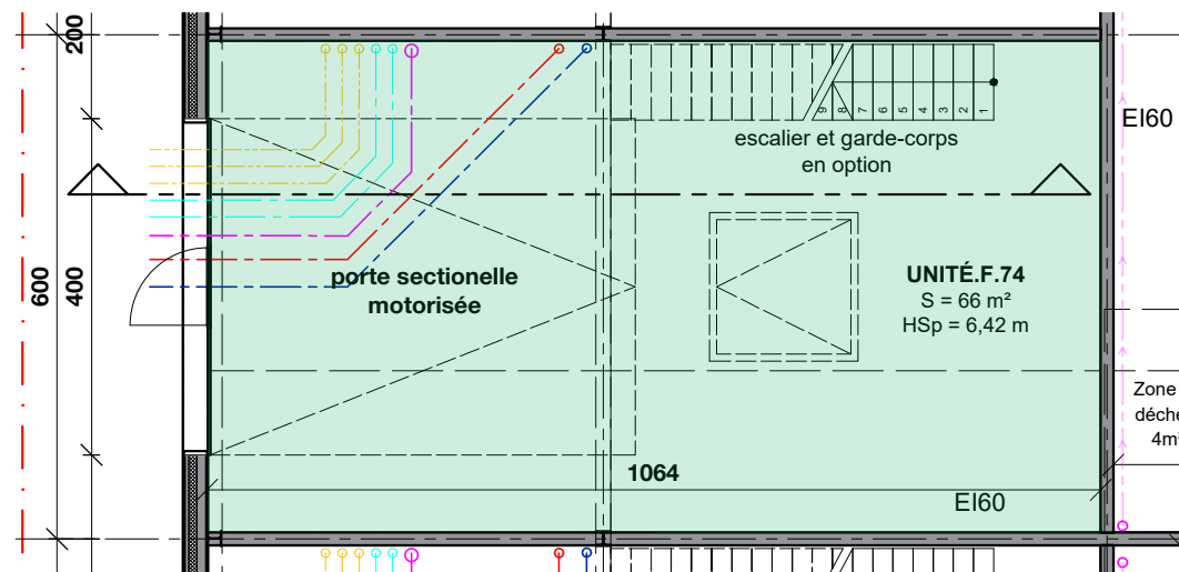
VUE EN PLAN RDC
