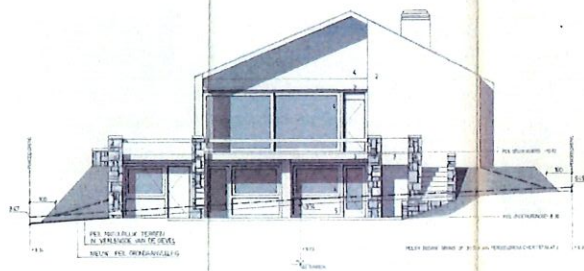
ACHTERGEVEL
