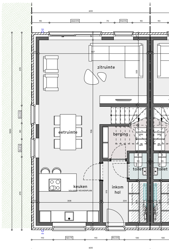
GRONDPLAN gelijkvloers
