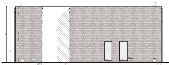
AANZICHT zijgevel
