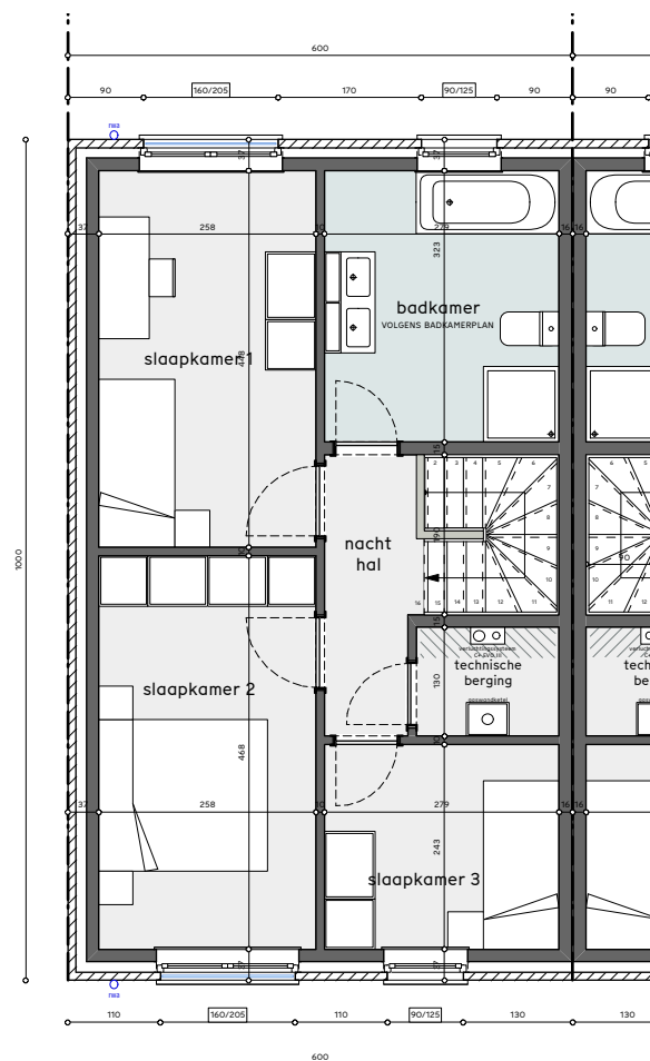
GRONDPLAN verdieping
