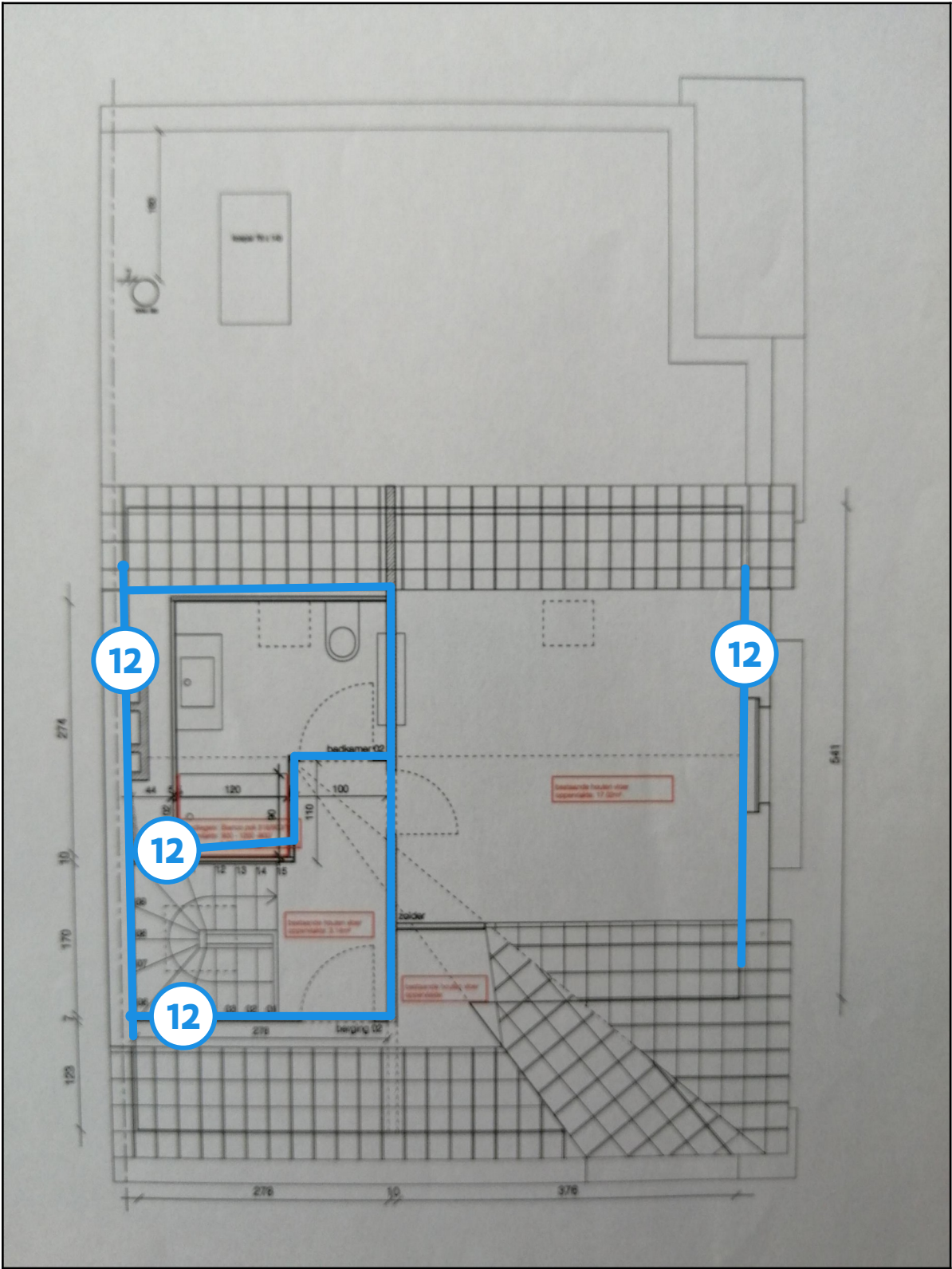
Legende van plan 1.10: gipsplan zolderverdieping
