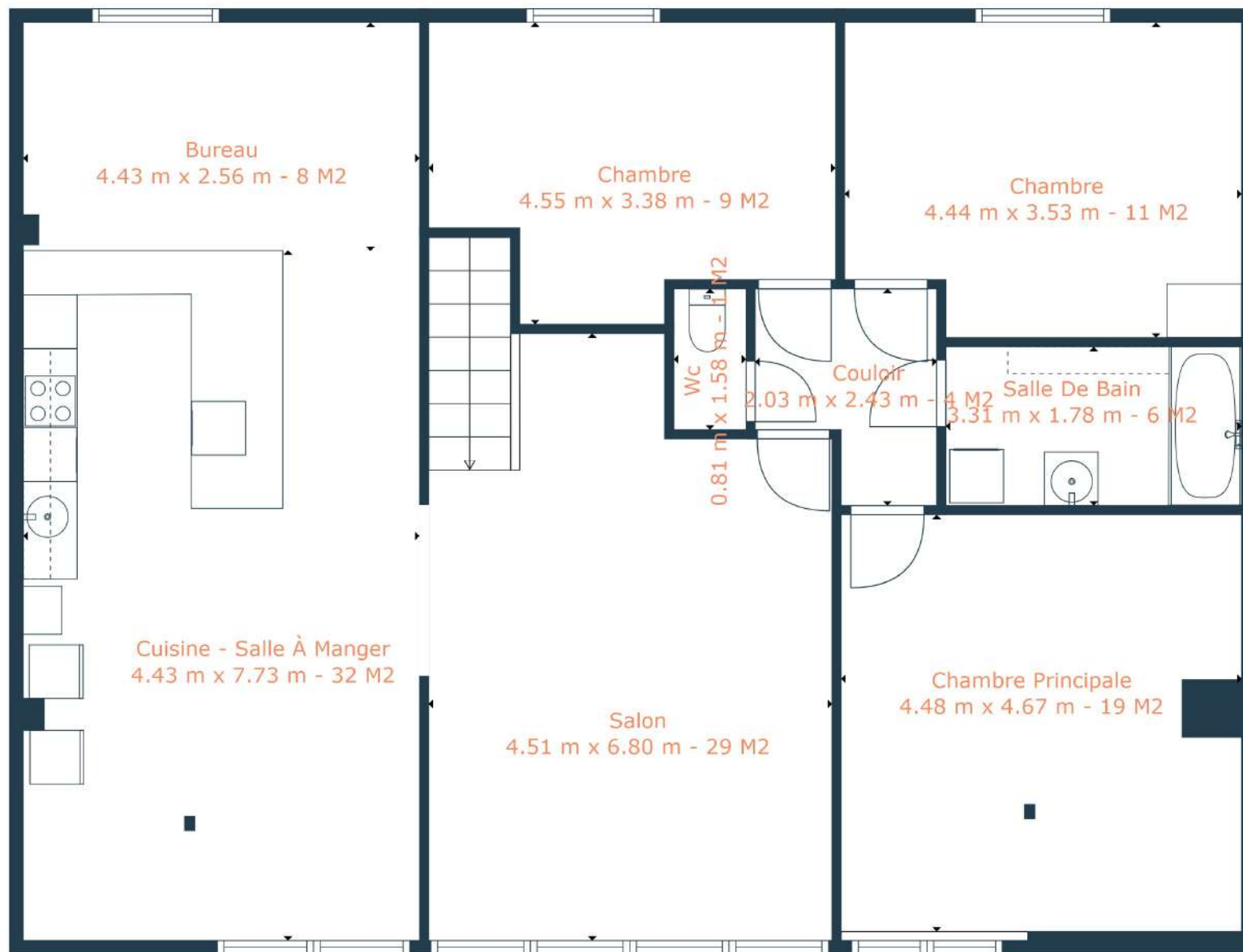
Étage 2
