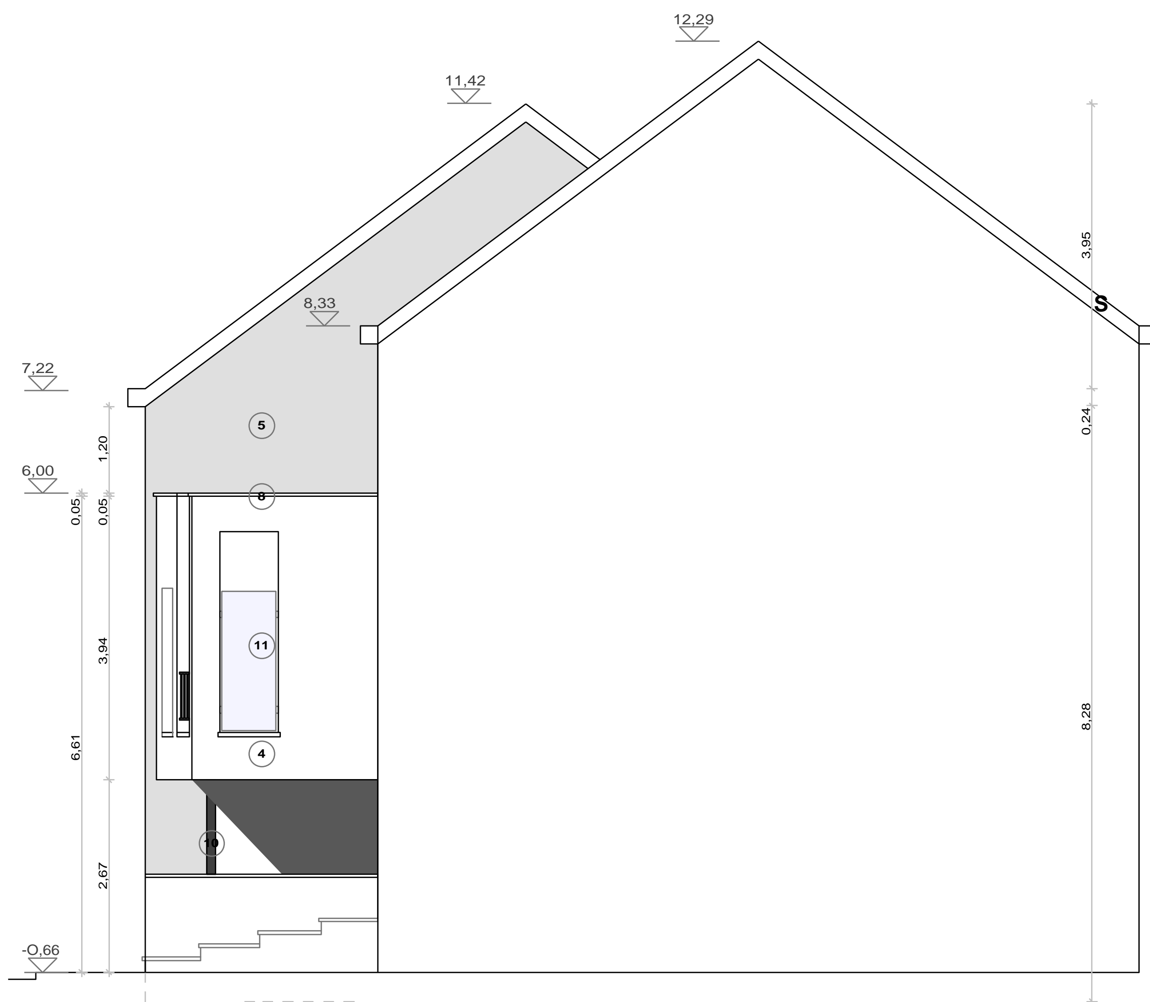
FACADE LATERALE DROITE
