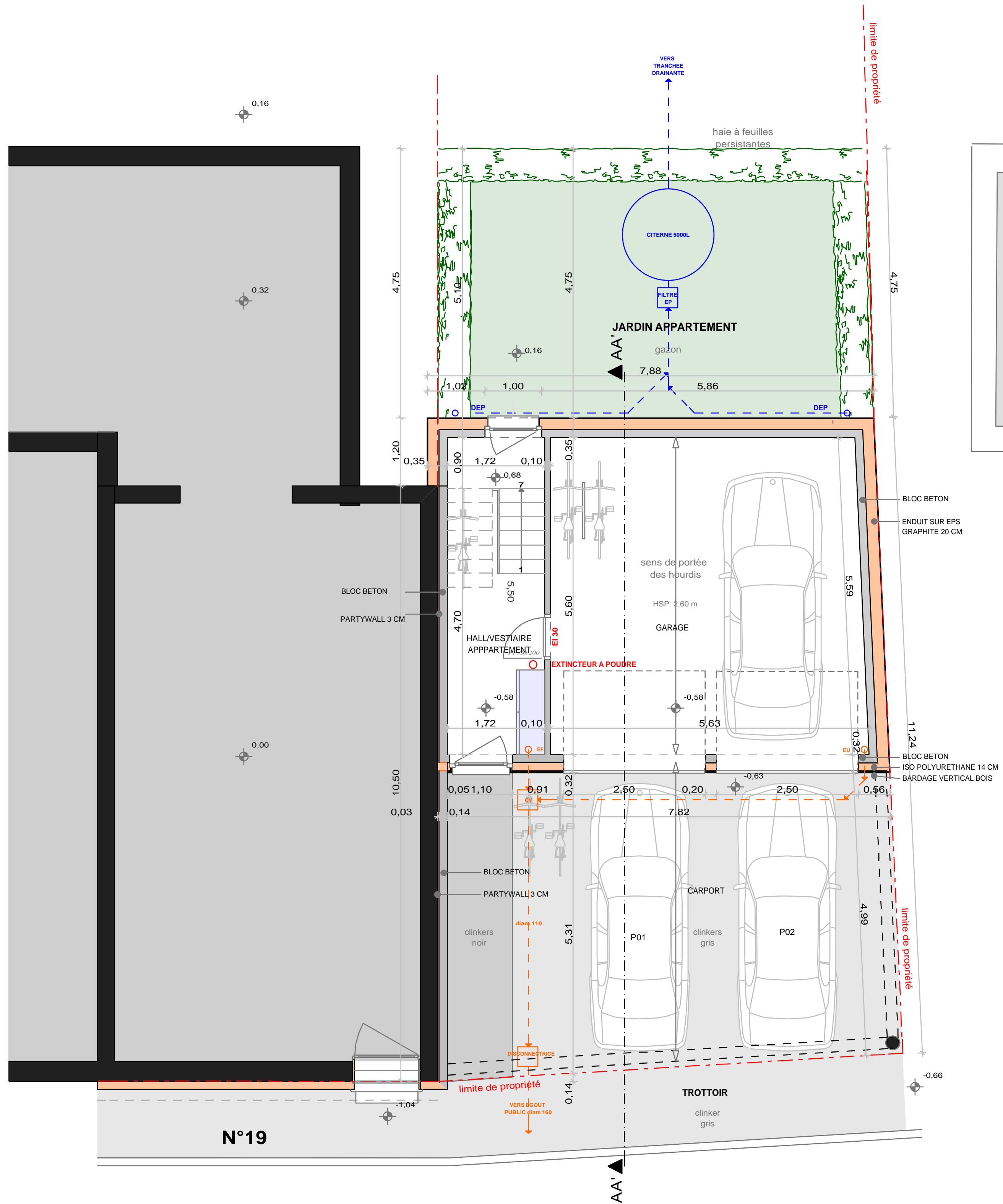
PLAN REZ-DE-CHAUSSEE
