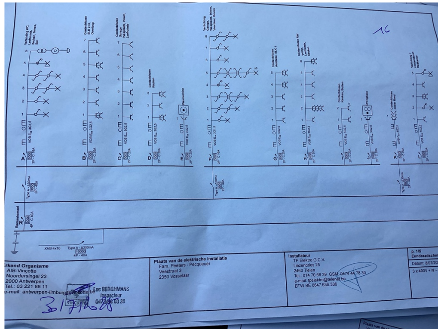
( Eendraadsschema's )
