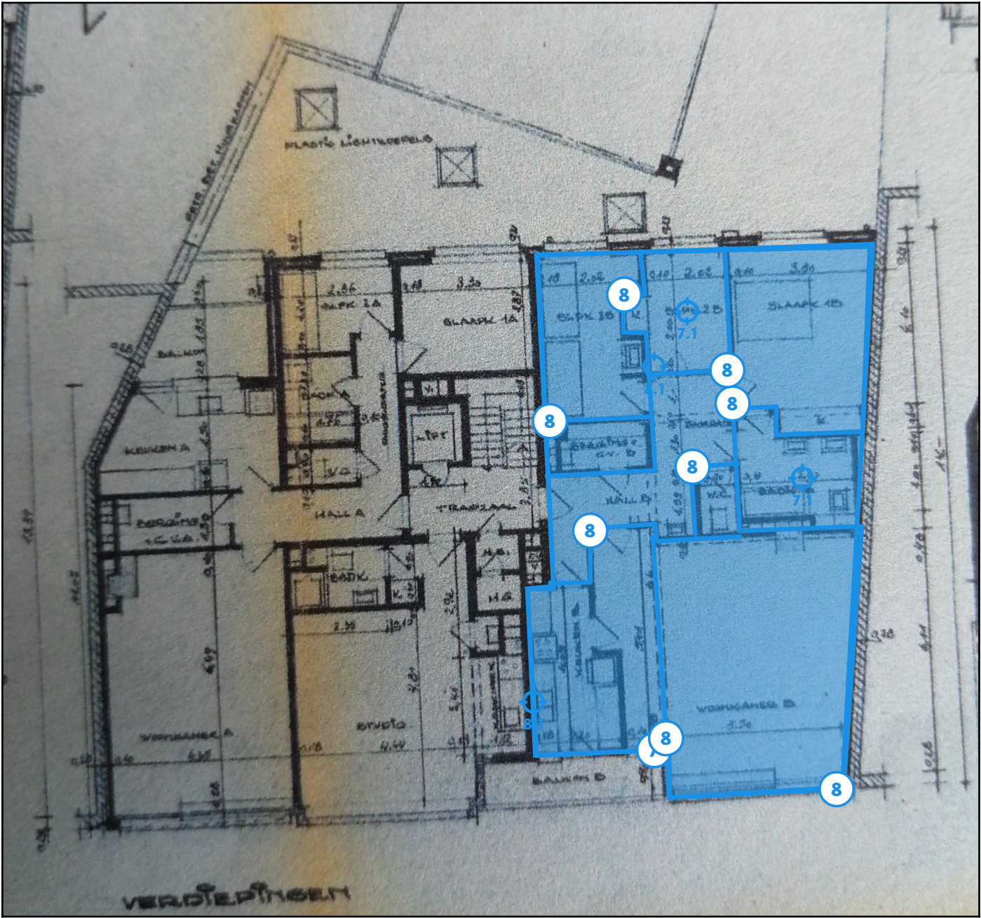
Legende van plan 1.2: gipsplan appartement
