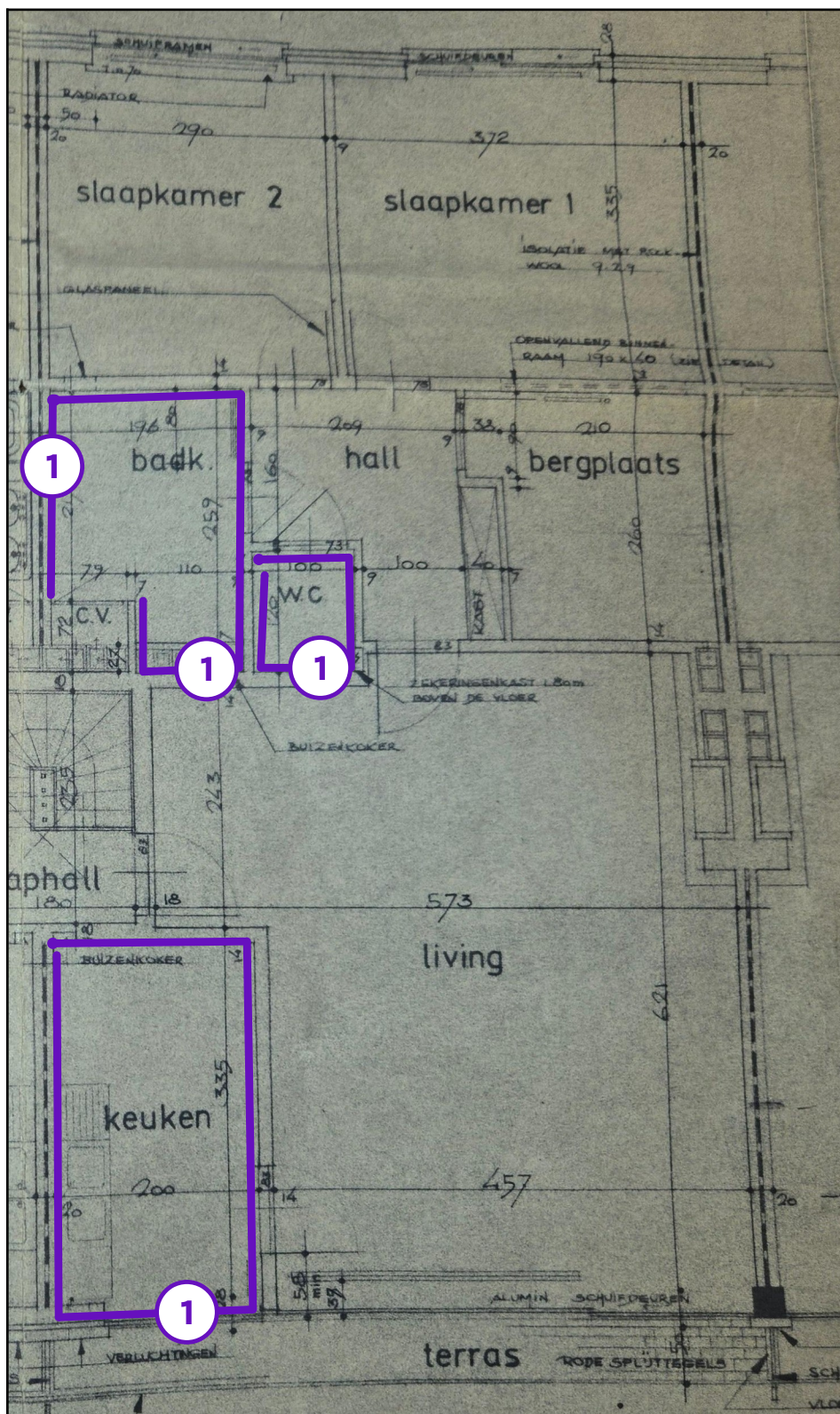
Legende van plan 1.2: Appartement B4
