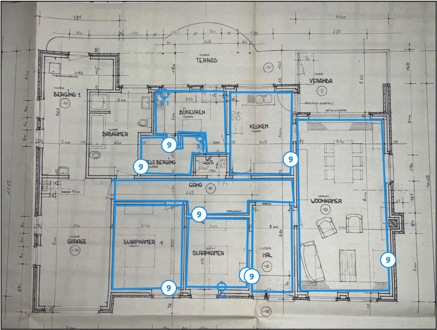
Legende van plan 1.1: Gelijkvloers woning
