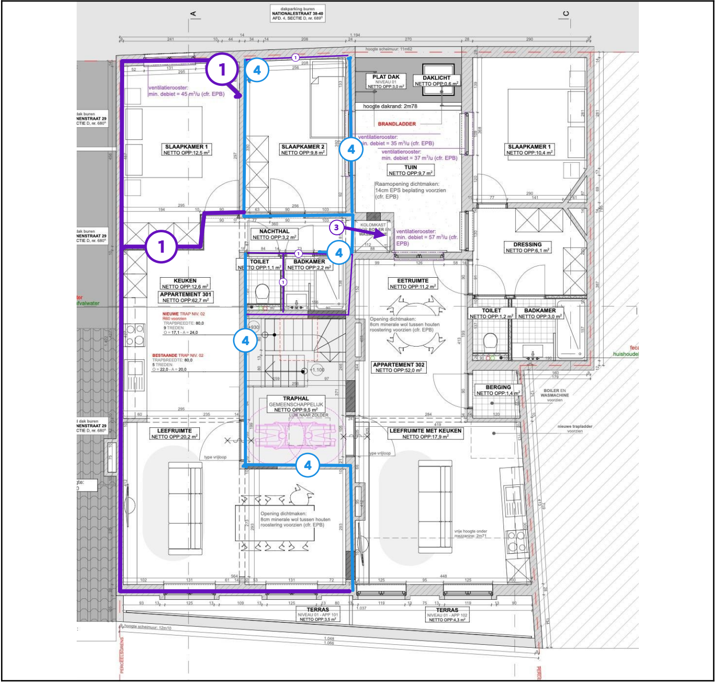
Legende van plan 1.1: Grondplan 3v
