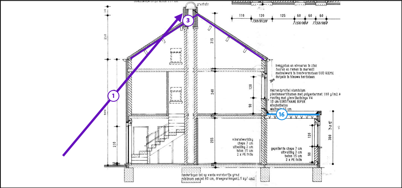
Legende van plan 1.4: doorsnede
