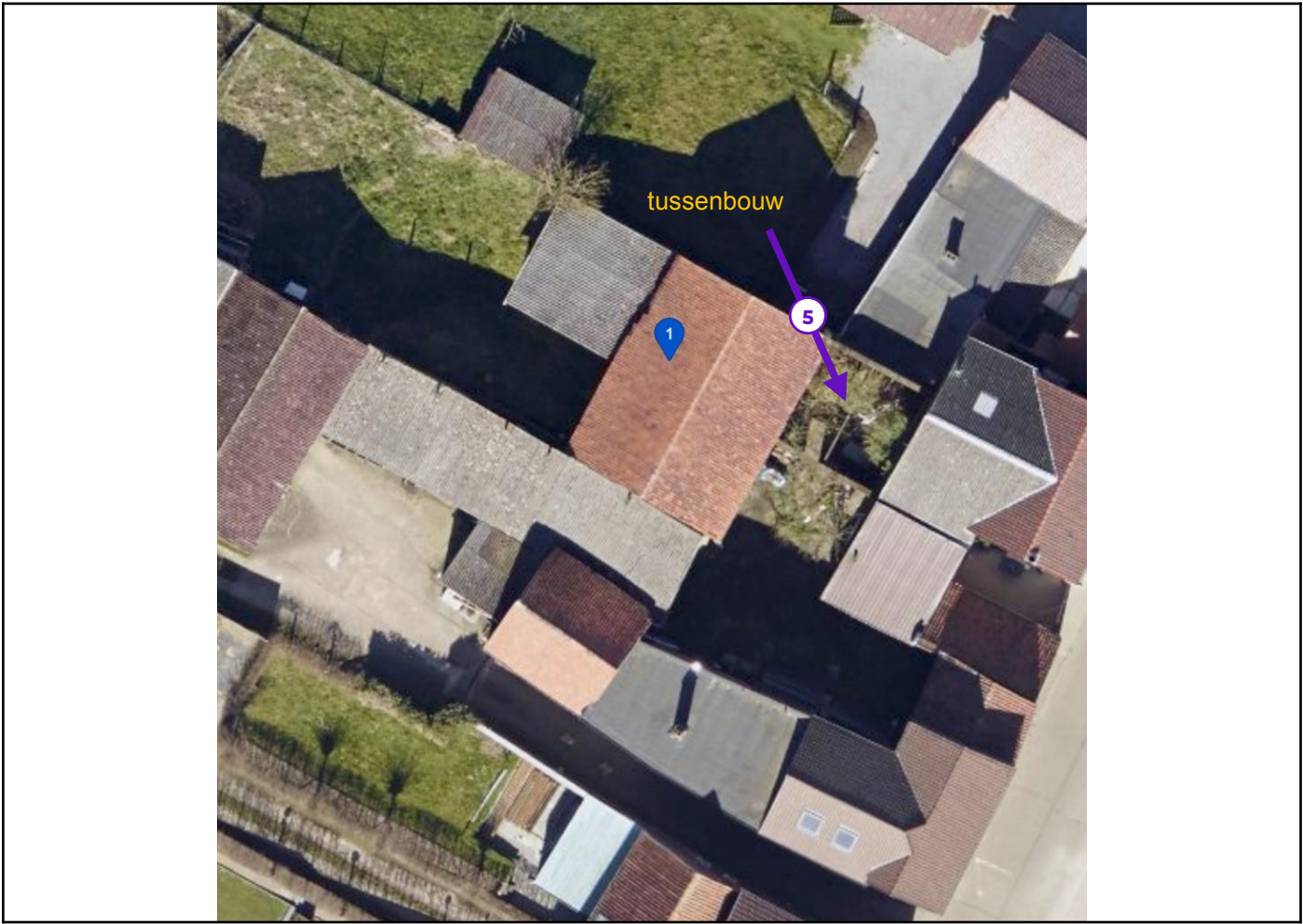
Legende van plan 4.2: sateliet foto 2015
