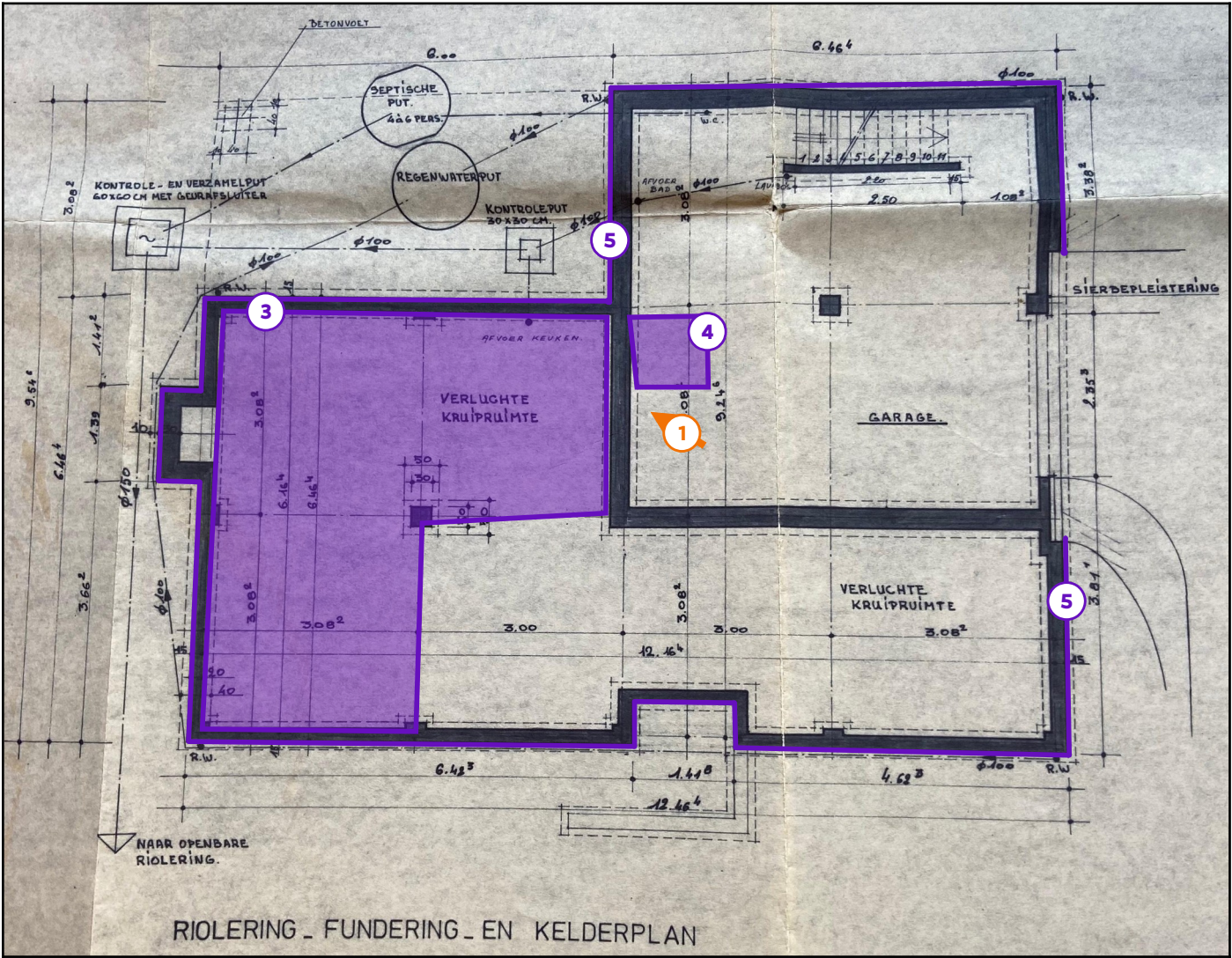
Legende van plan 1.3: kelder + garage
