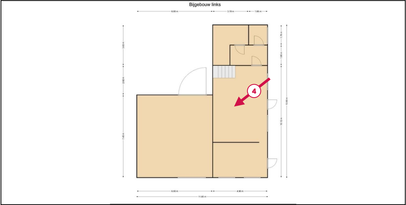
Legende van plan 1.8: Plan bijgebouw links - VD1
