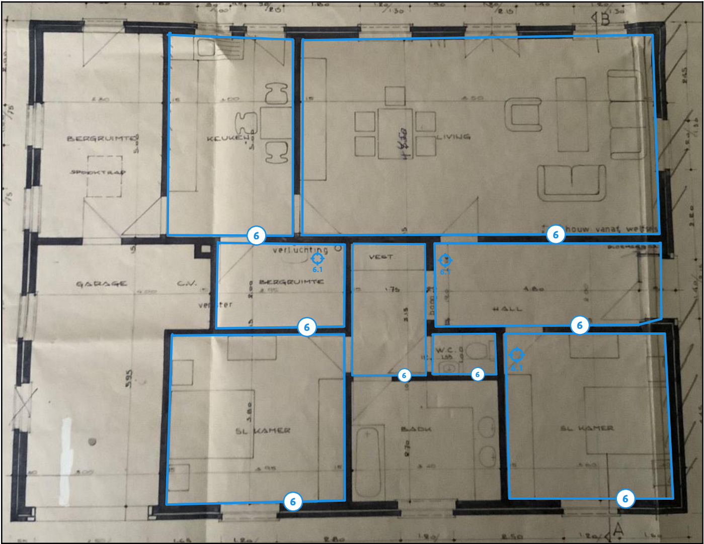
Legende van plan 1.2: Gelijkvloers - pleisterwerk wanden
