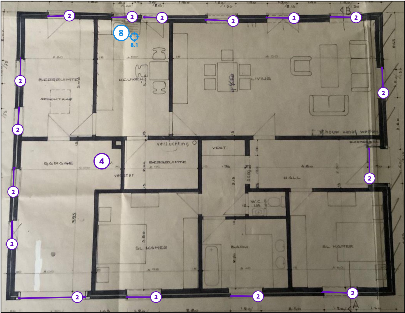
Legende van plan 1.1: Gelijkvloers - silicone - anti dreun - cv ketel
