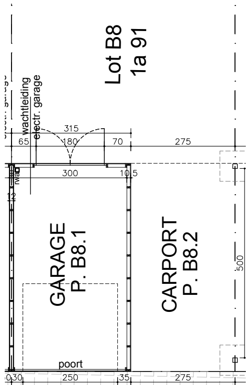
grondplan carport/garage B8
