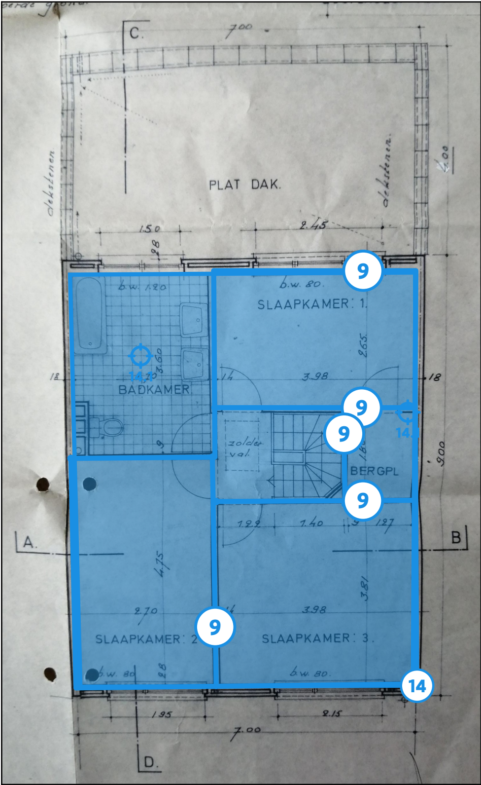
Legende van plan 1.6: gipsplan verdieping
