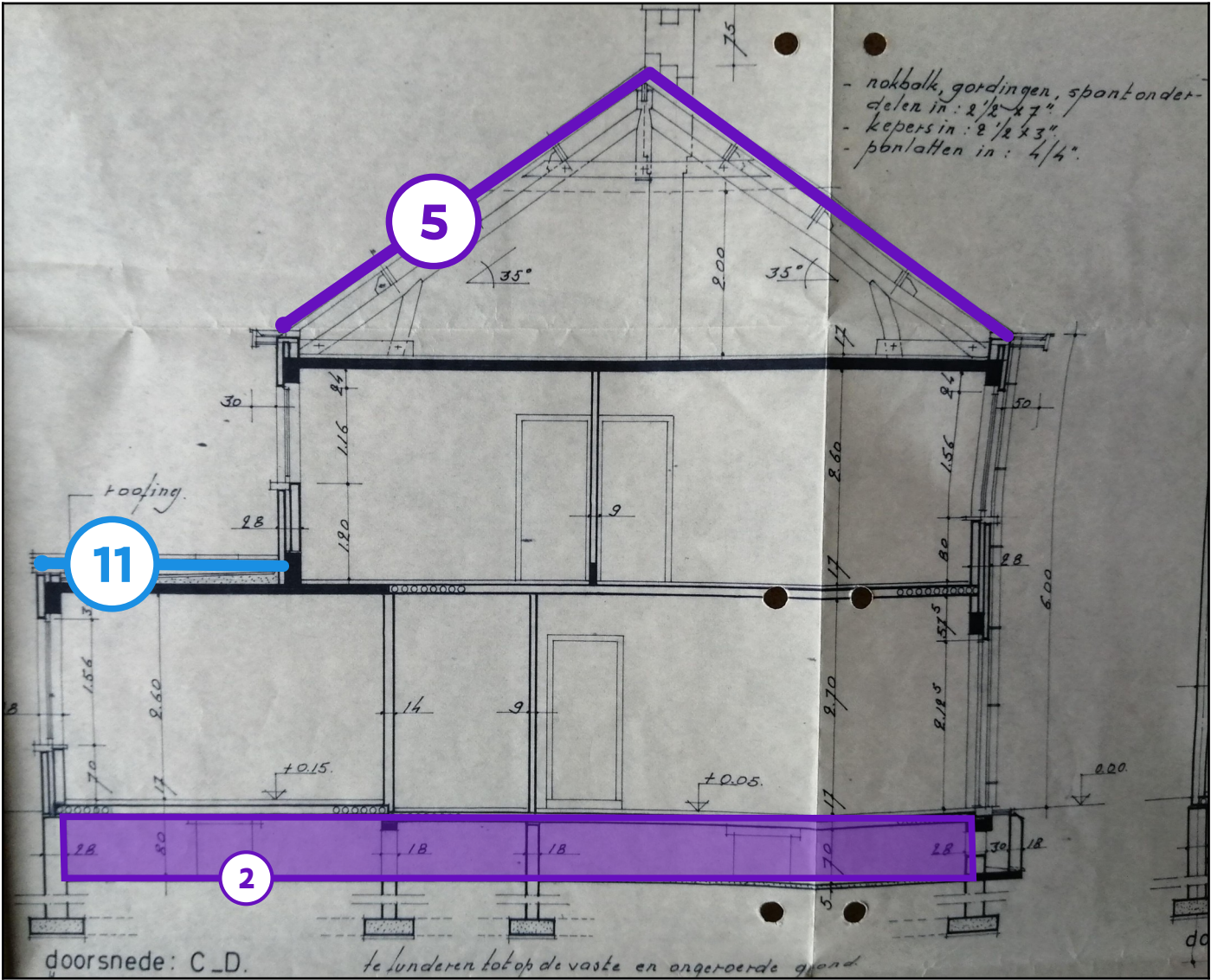
Legende van plan 1.9: snede C-D
