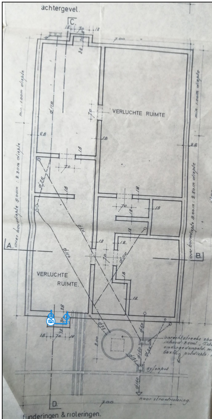
Legende van plan 1.1: fundering
