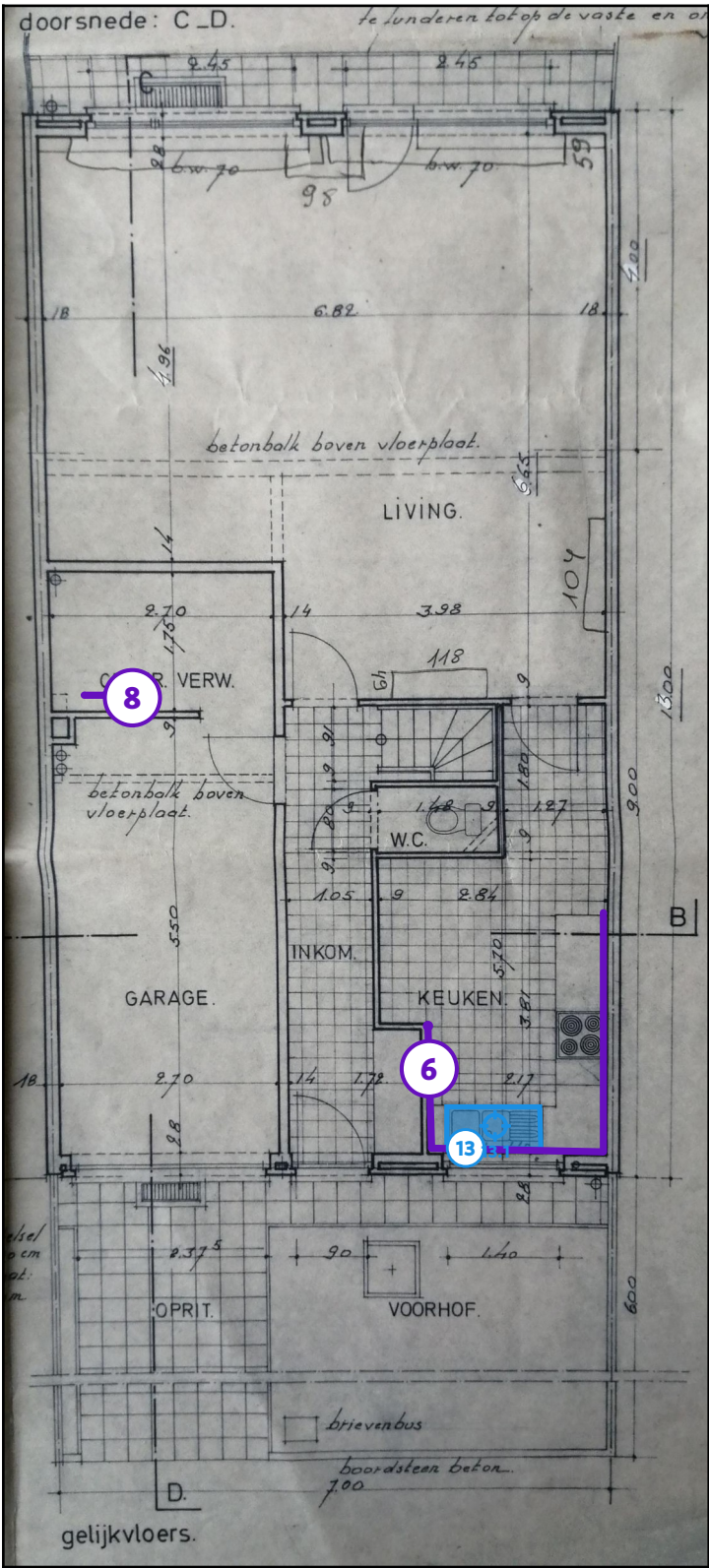
Legende van plan 1.2: grondplan gelijkvloers
