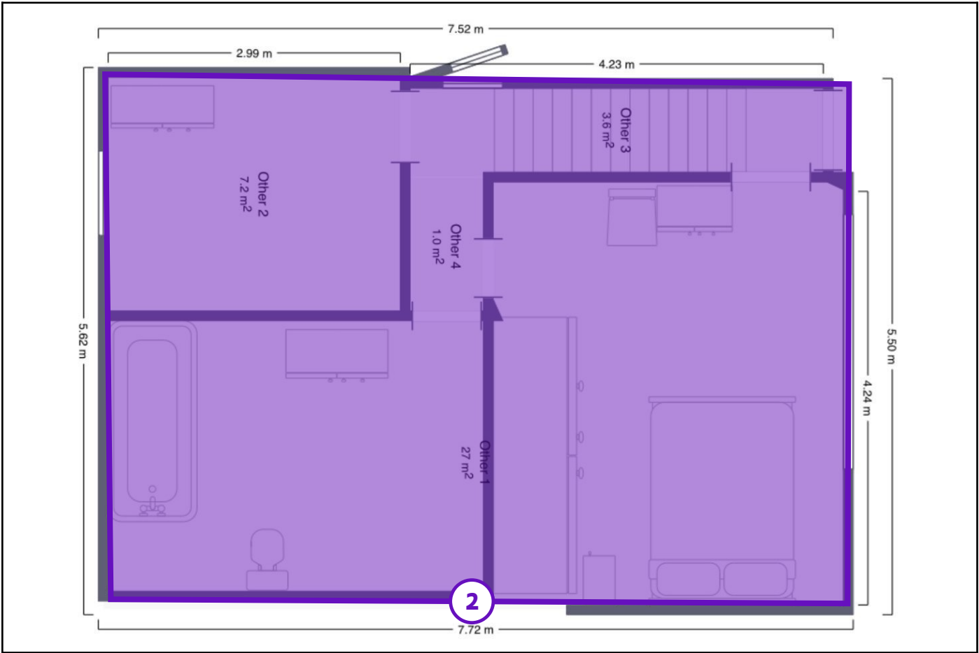
Legende van plan 1.4: Grondplan 1v
