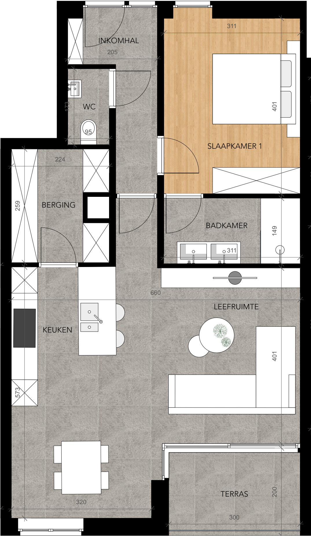
SCHAAL: 1/50
