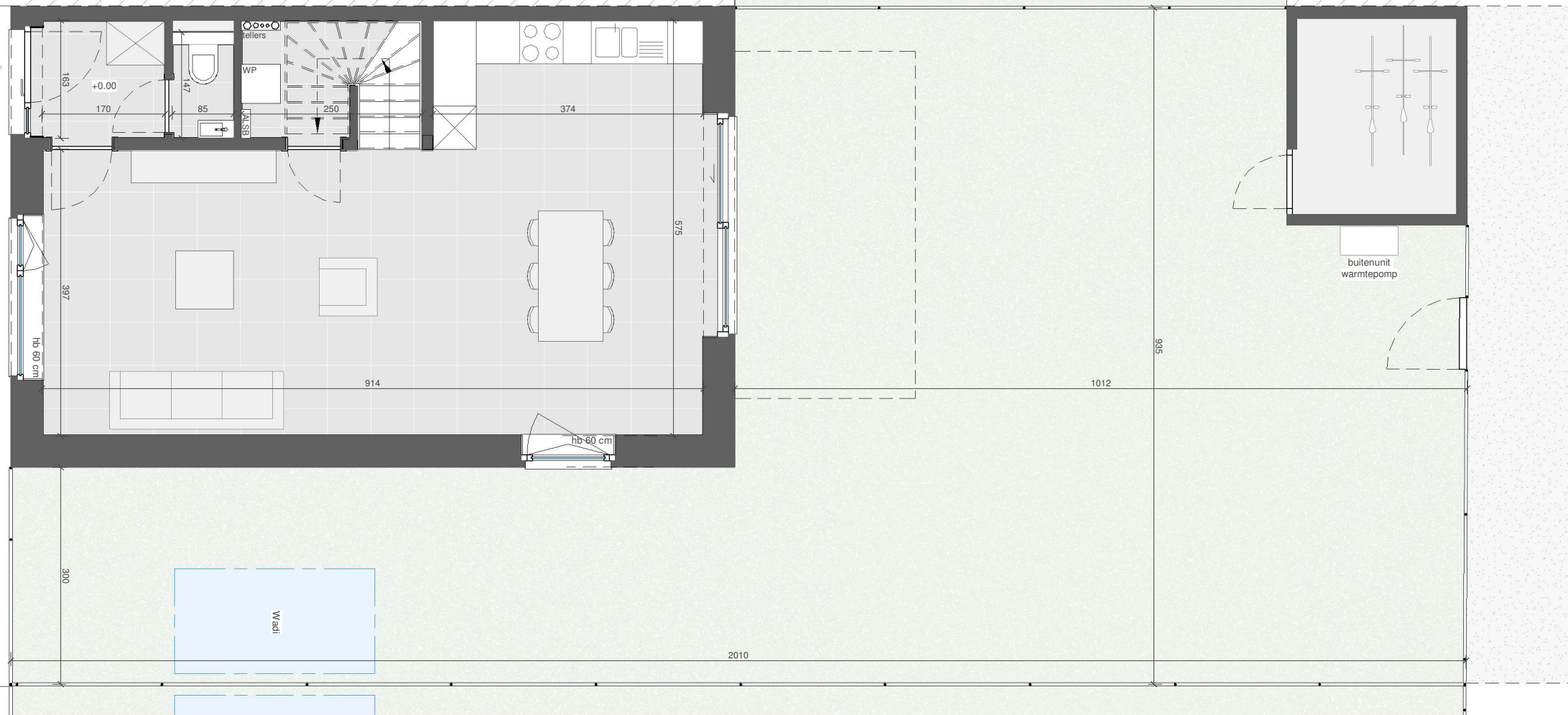
GELIJKVLOERS
