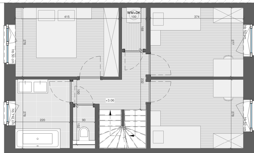
VERDIEPING
