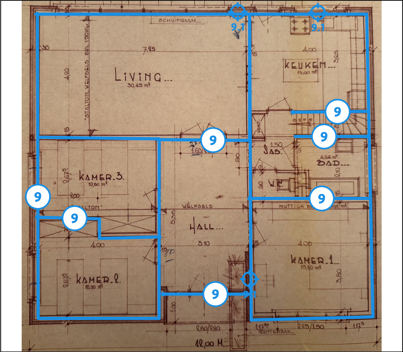
Legende van plan 1.1: Plan gelijkvloers
