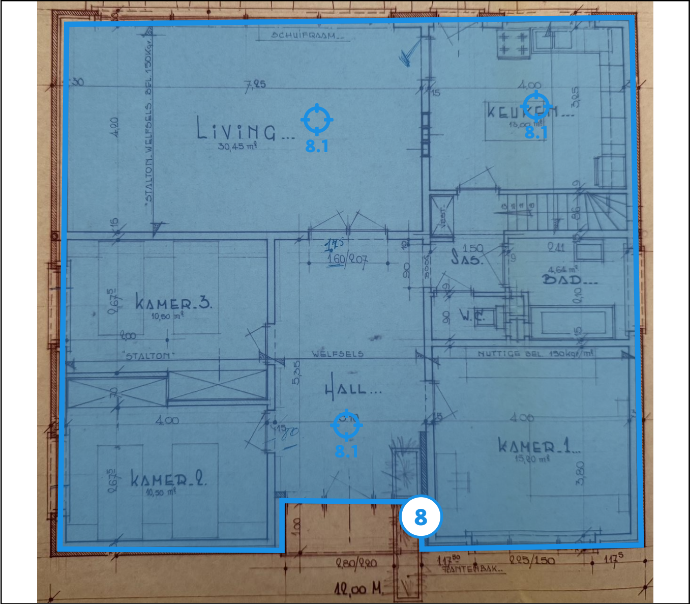
Legende van plan 1.3: Plan gelijkvloers
