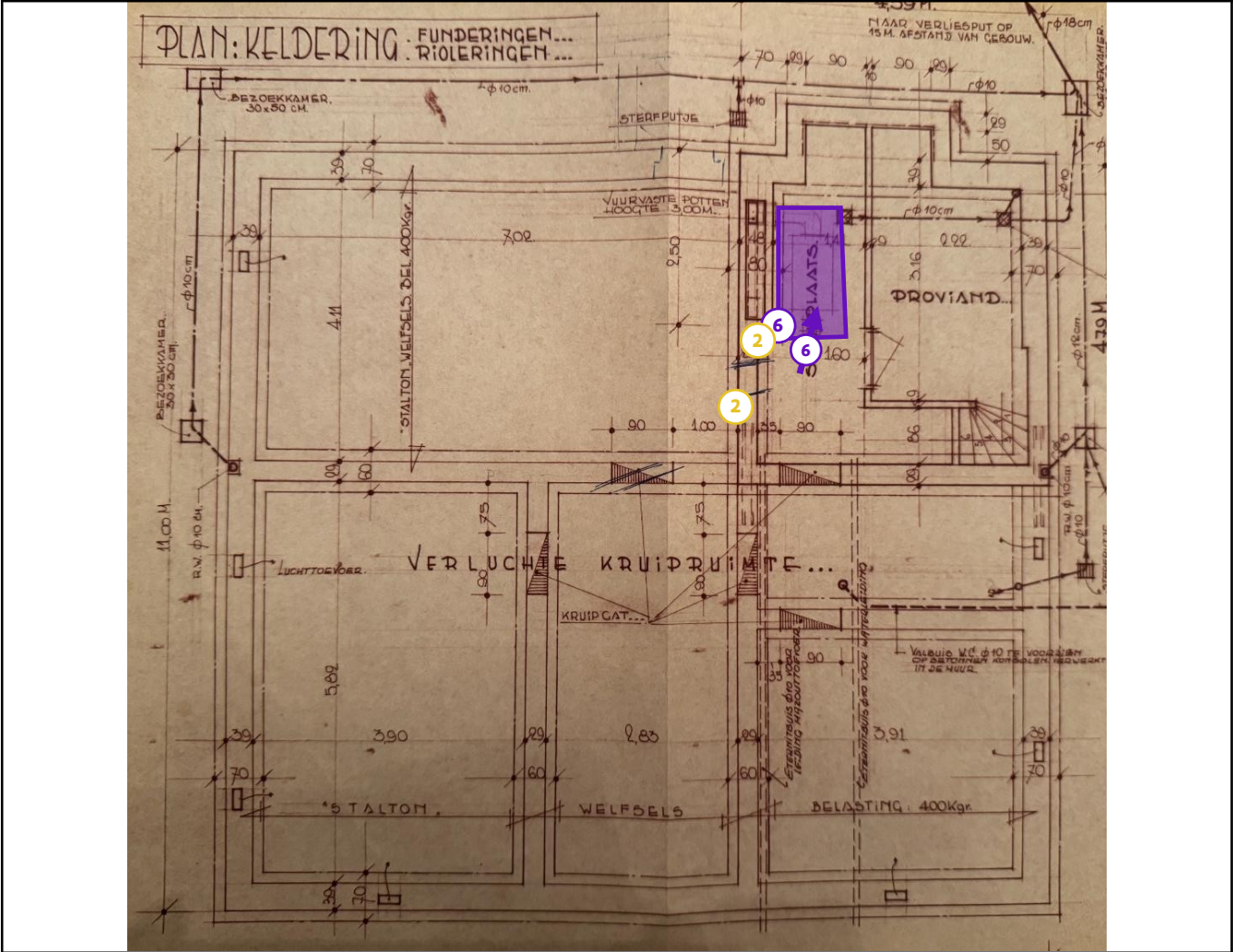
Legende van plan 1.6: Plan kelder
