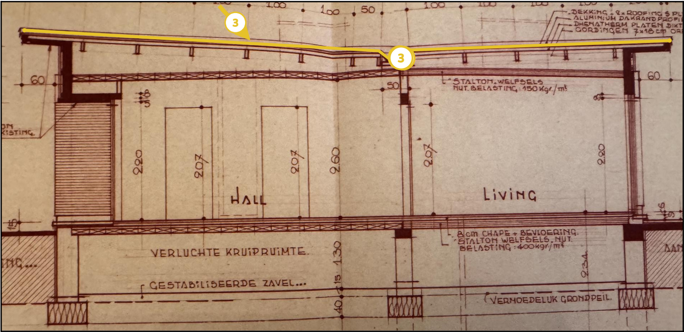
Legende van plan 1.5: Plan doorsnede
