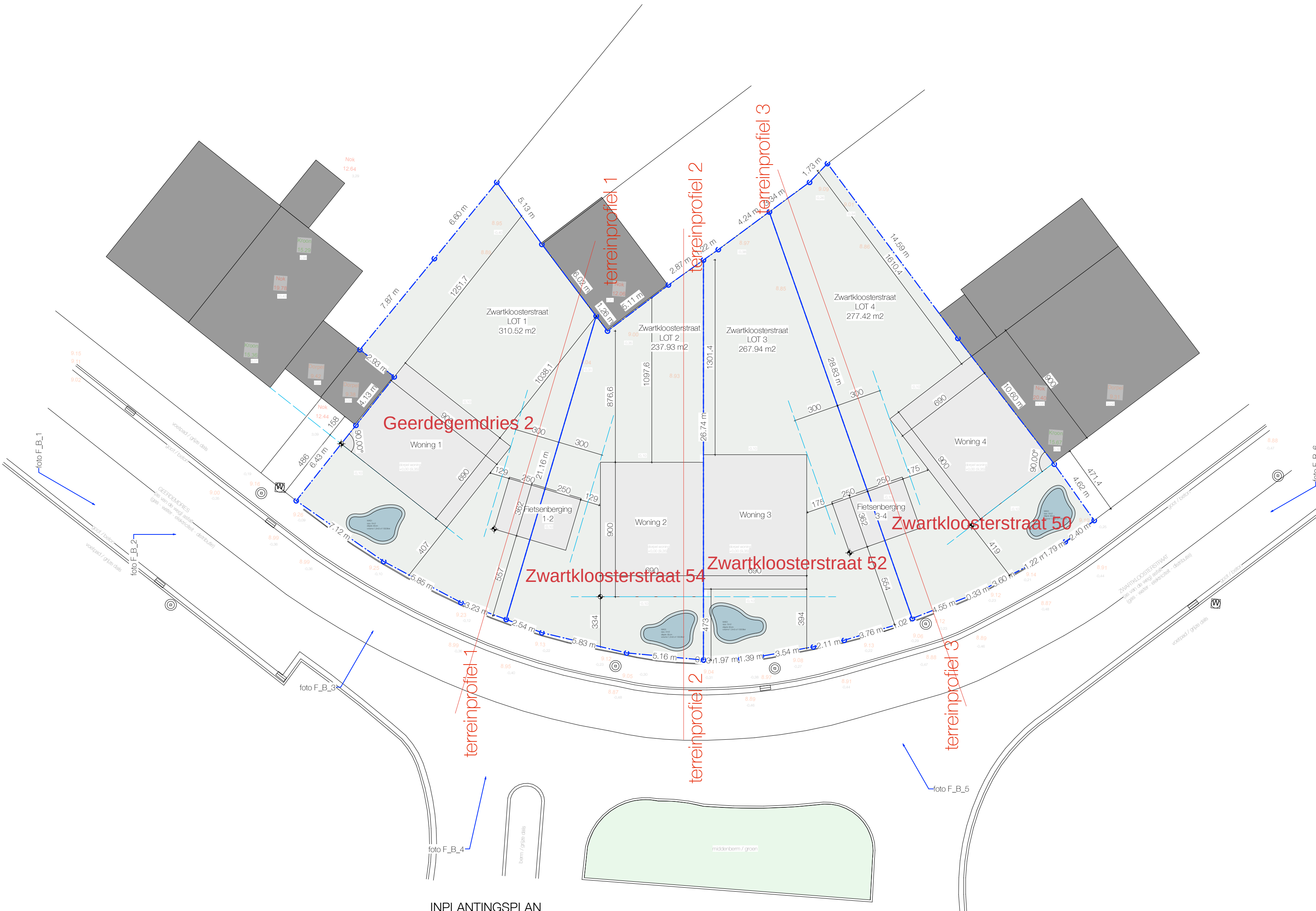
INPLANTINGSPLAN Schaal: 1:200
