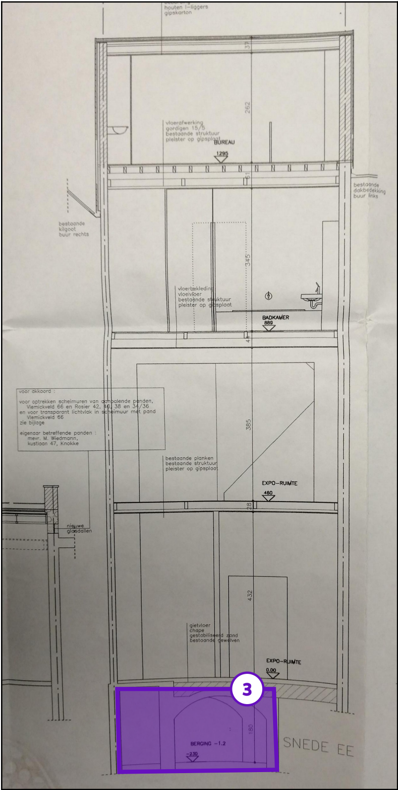
Legende van plan 1.10: snede EE
