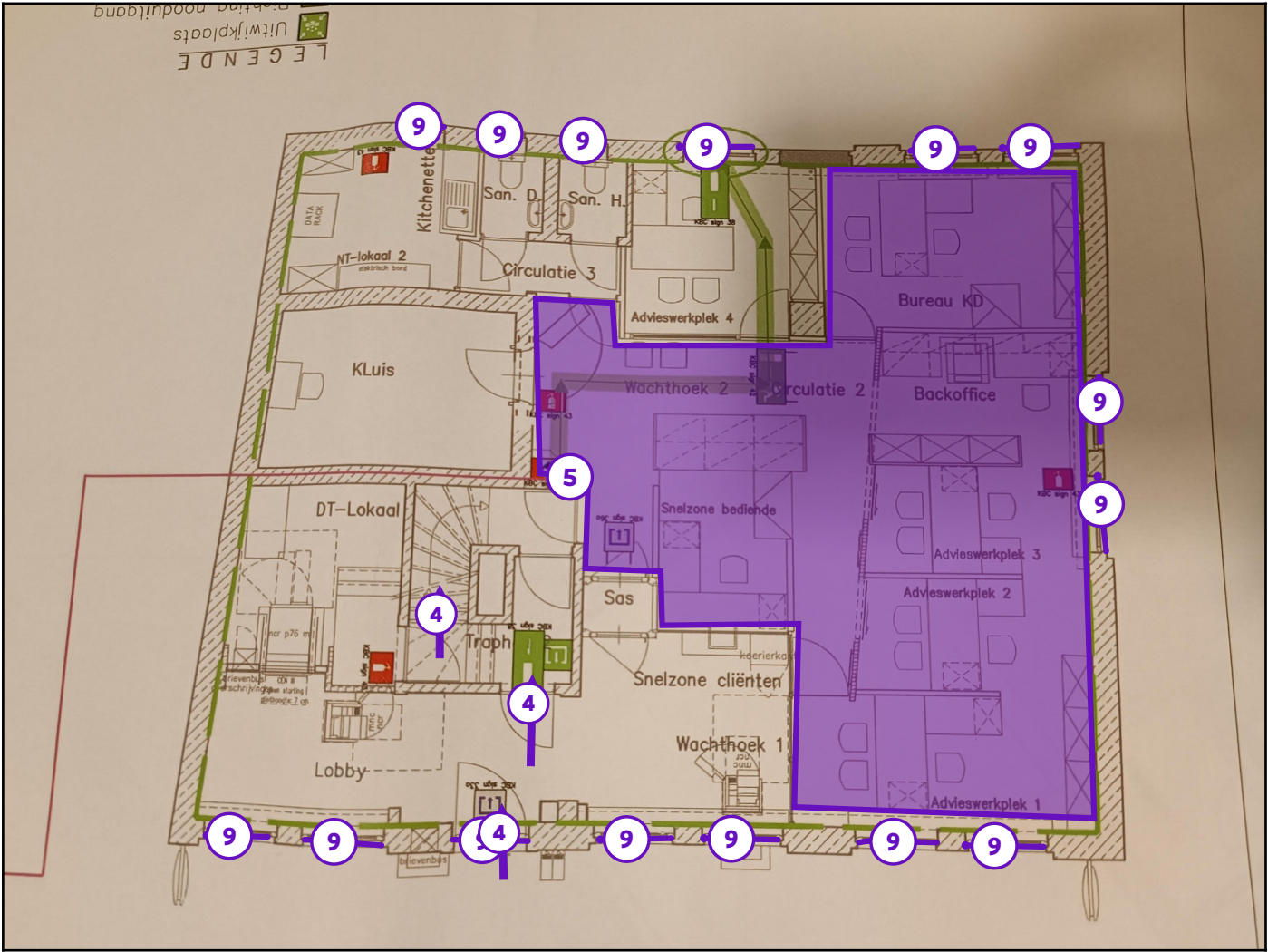
Legende van plan 1.9: Gelijkvloers
