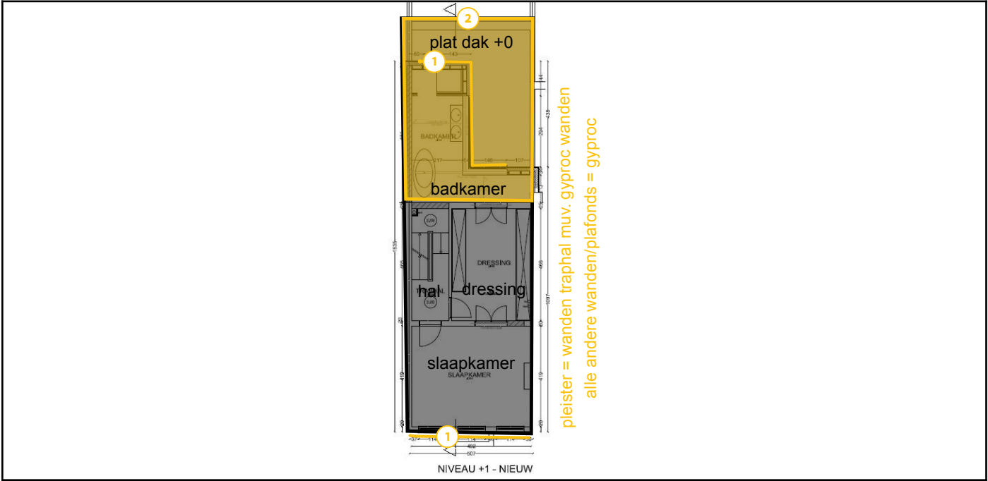
Legende van plan 1.3: Hoofdgebouw plan +1
