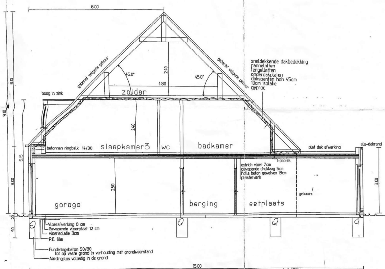
DOORSNEDEN AB
