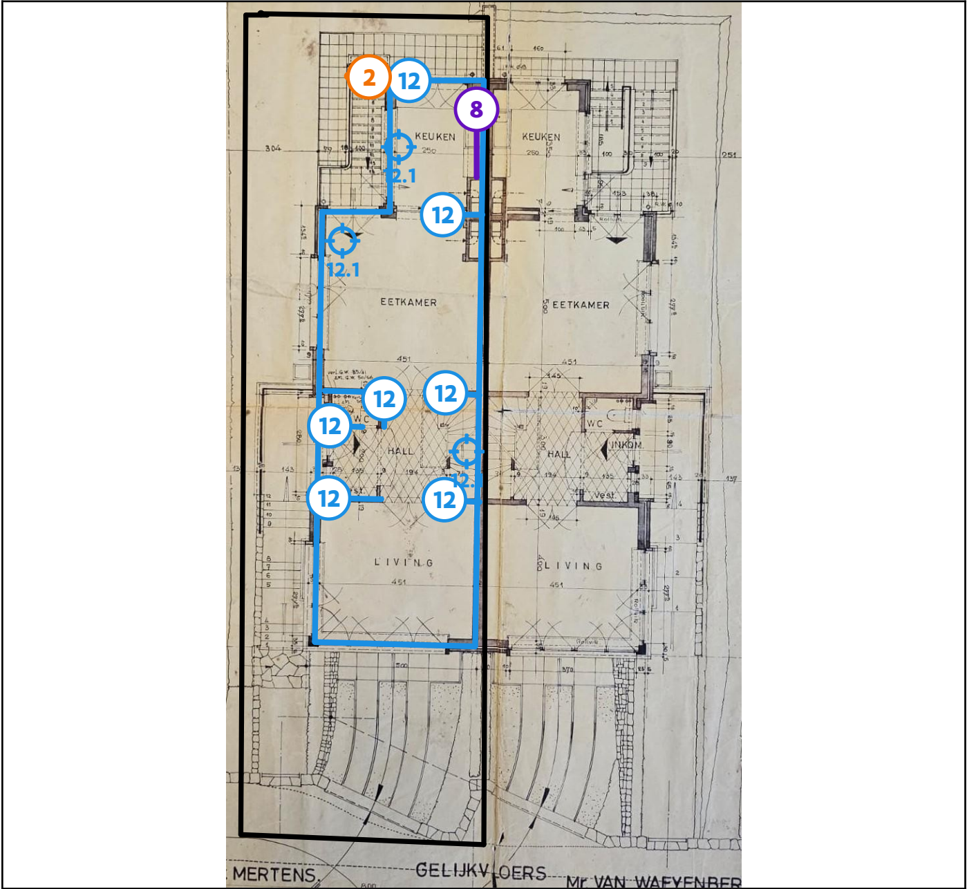
Legende van plan 1.6: Plan gelijkvloers
