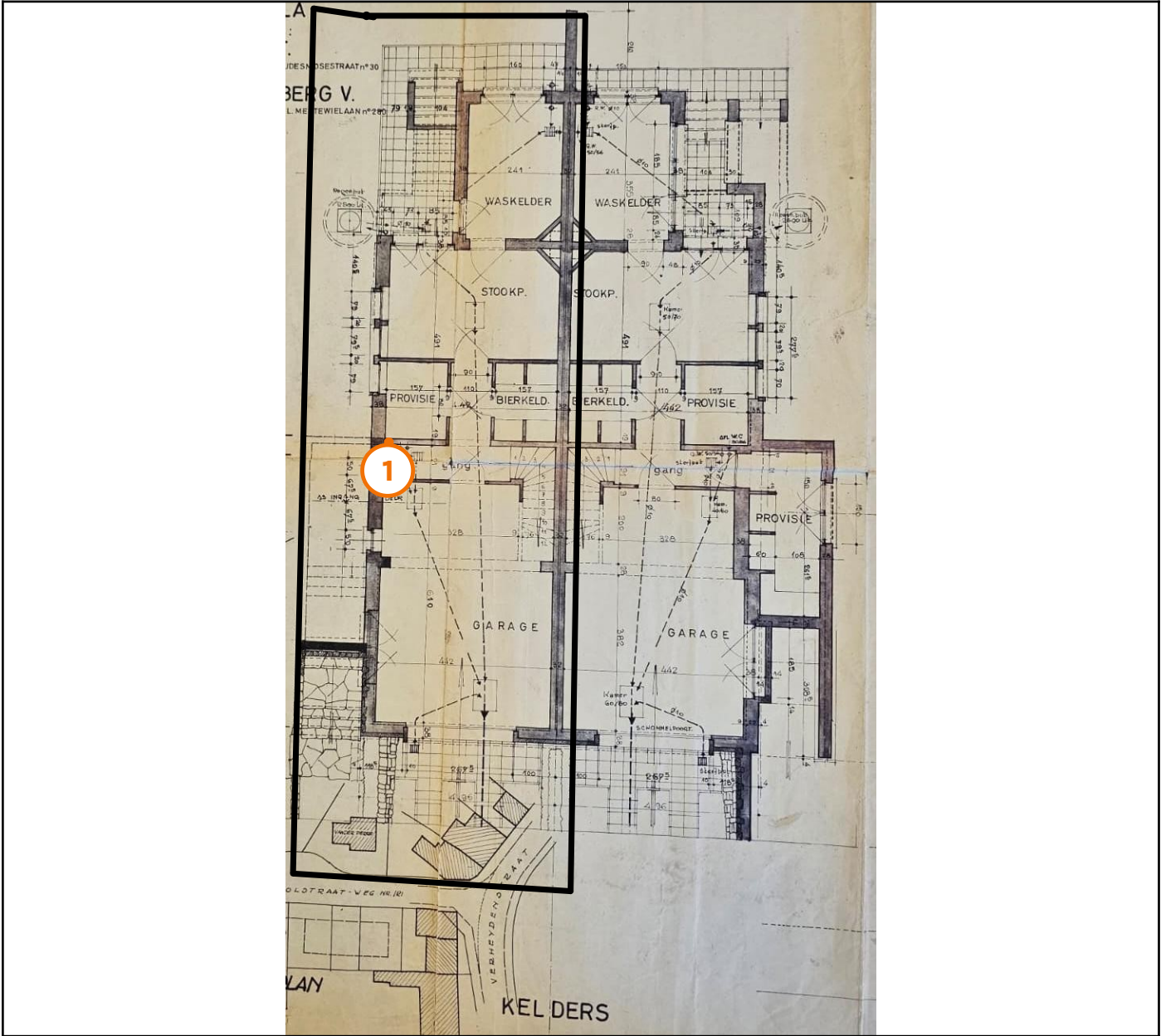
Legende van plan 1.5: Plan kelder
