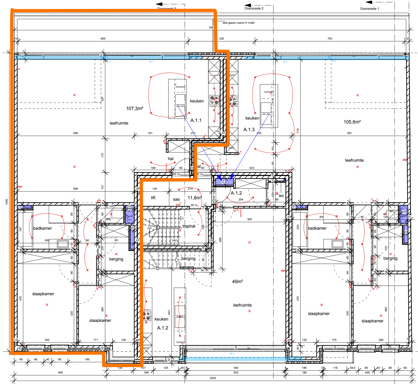
VERDIEPING 1 schaal 1/100
