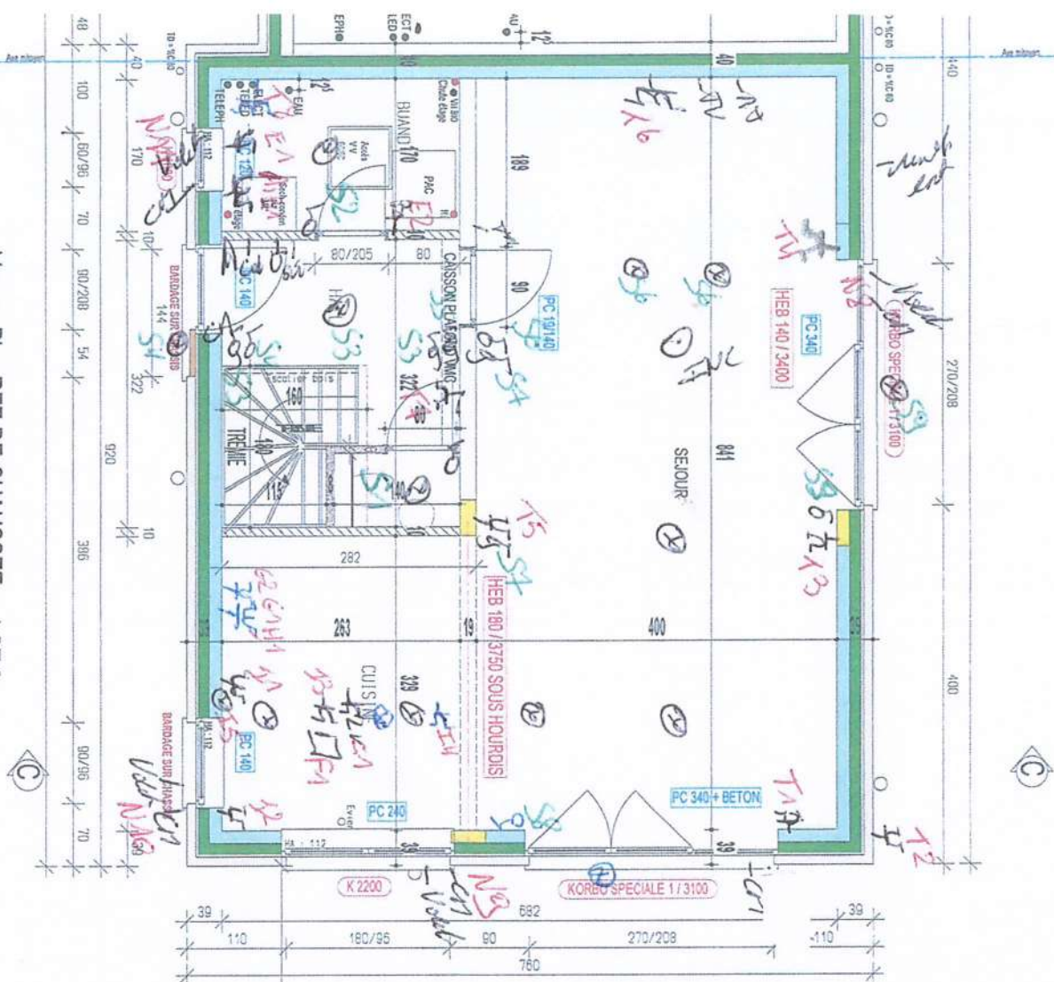
Vue en Plan REZ-DE-CHAUSSEE LOT 3
