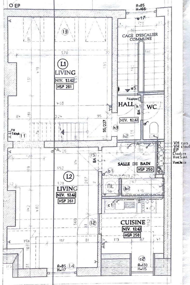
NIVEAU R+3 (AP.IV)
