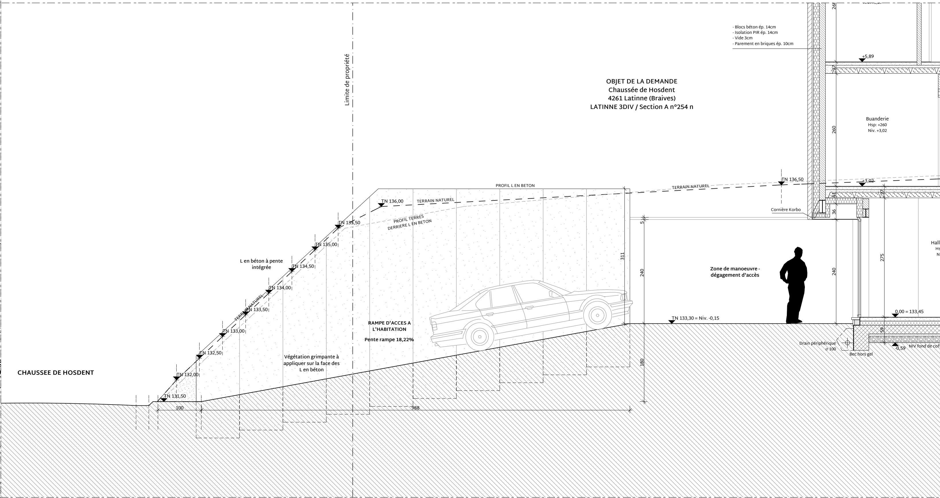
Coupe allée d'accès - vue latérale gauche - 1/50
