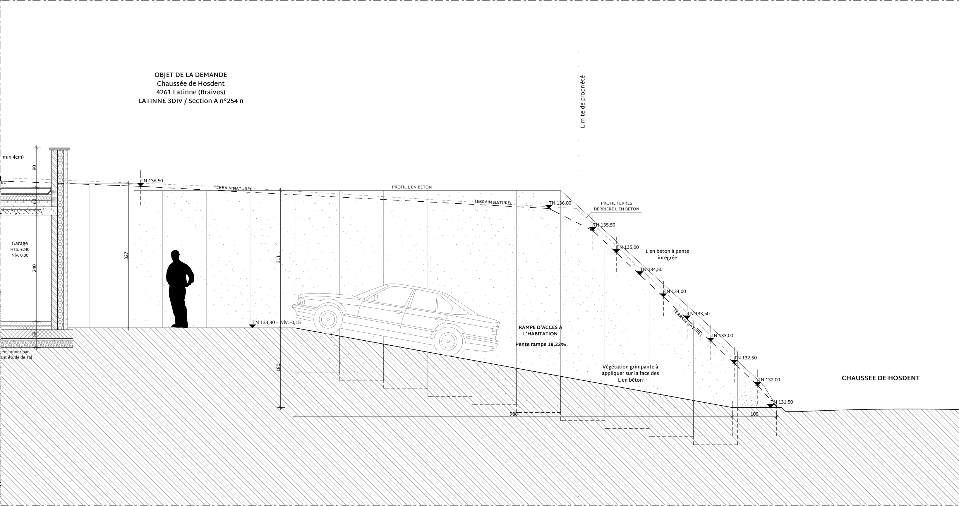
Coupe allée d'accès - vue latérale droite - 1/50
