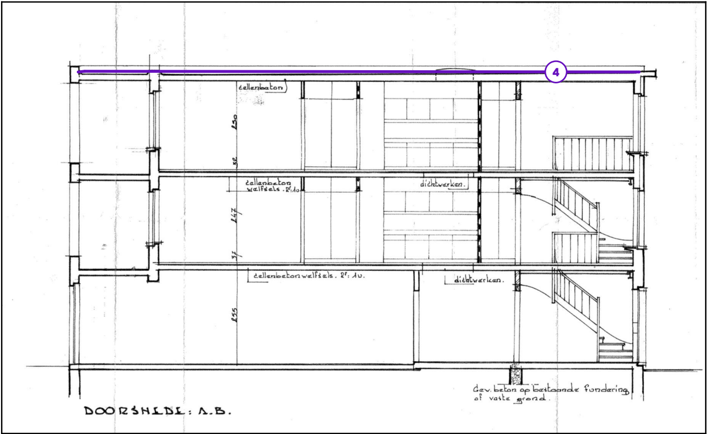
Legende van plan 1.4: Doorsnede
