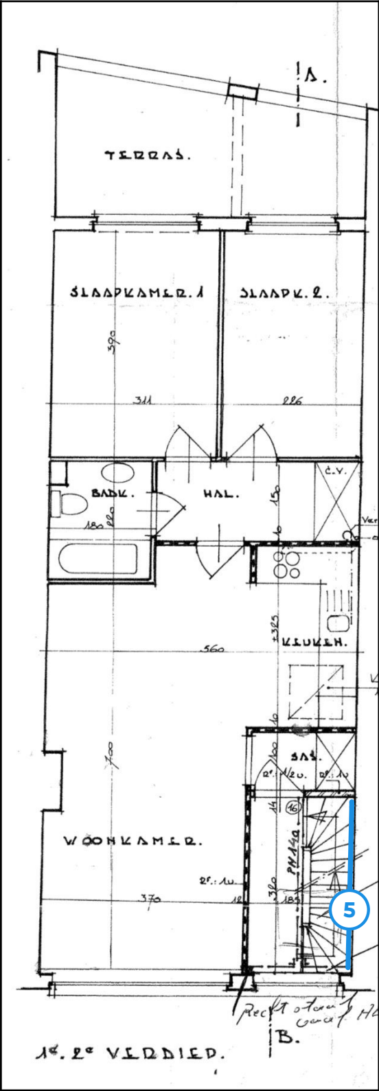
Legende van plan 1.2: 1ste verdieping
