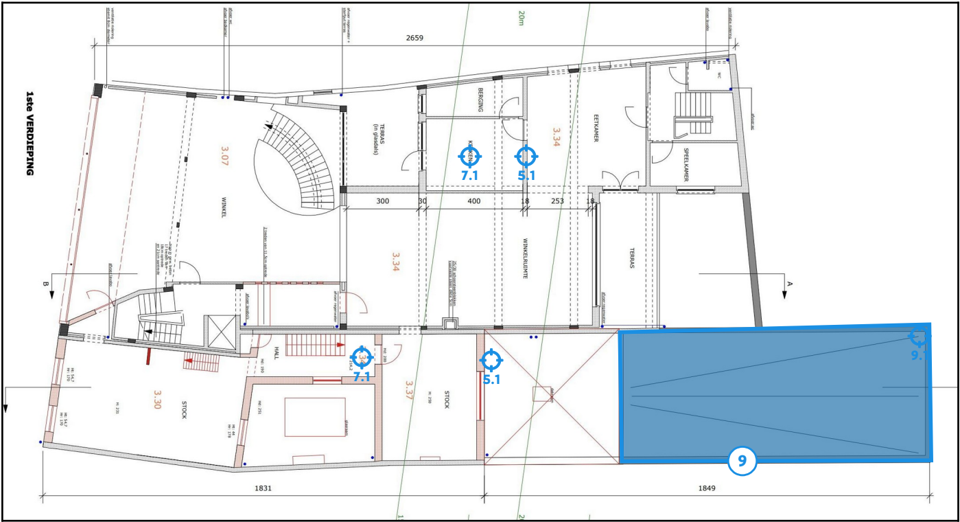
Legende van plan 1.3: 1ste verdieping langensteenweg 5 Merchtem
