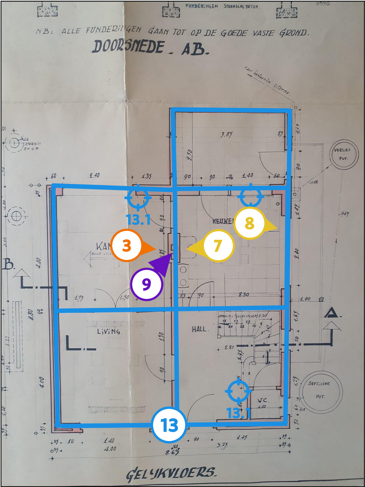
Legende van plan 1.2: gelijkvloers (muren)
